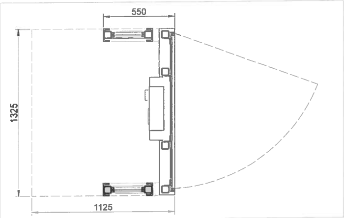
01 Plan
