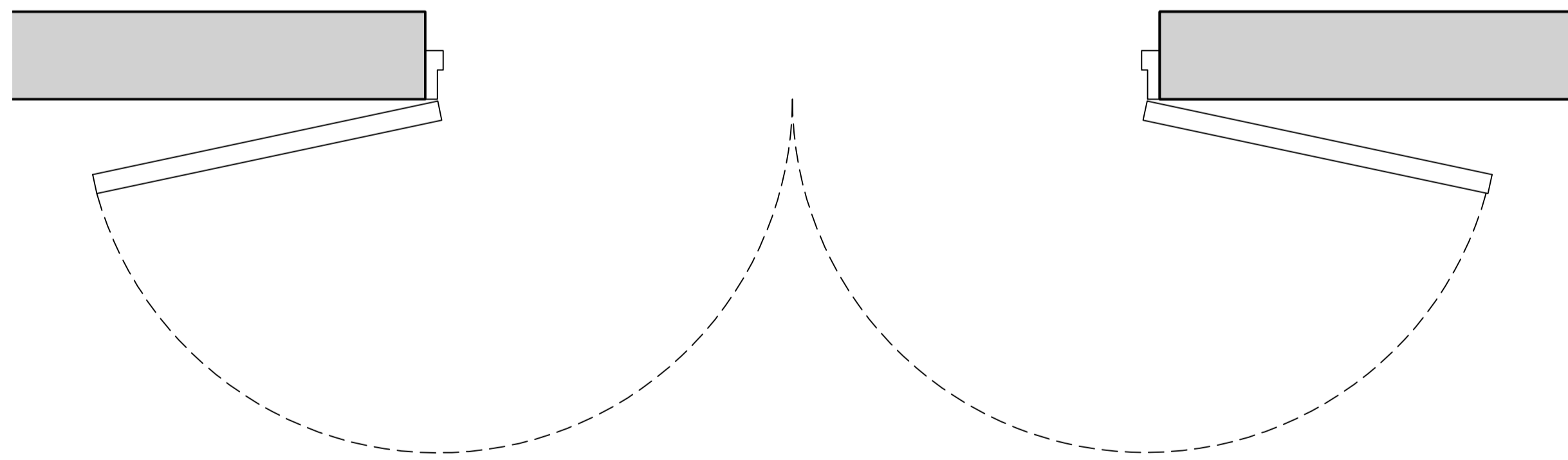
Door type C Section Four paneled double hinged door 00.03 Door type C Internal double hinged door
