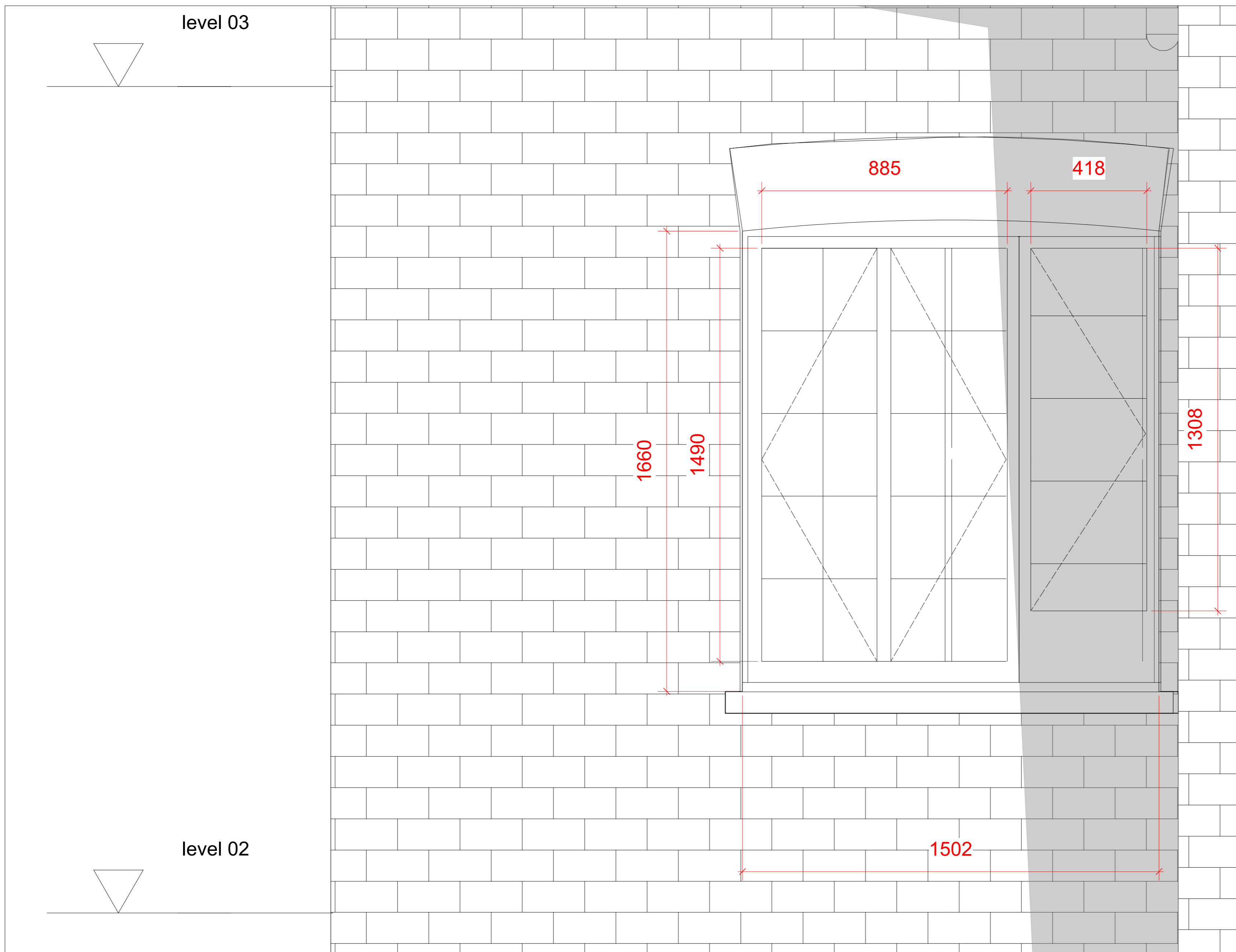
1 EXISTING ELEVATION 02 Scale: 1:10
