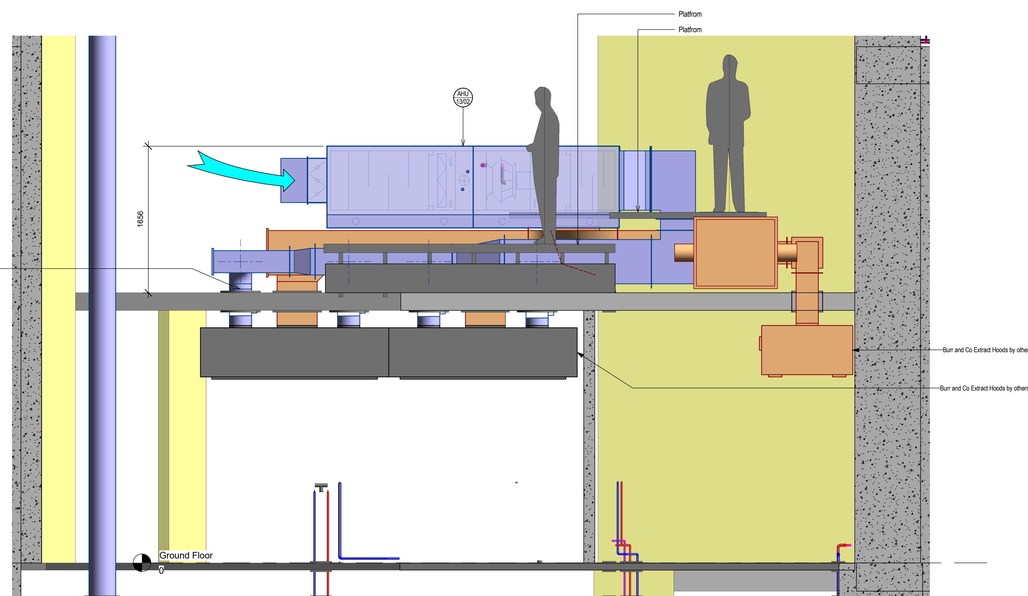
2 Section A - A 1 : 25
