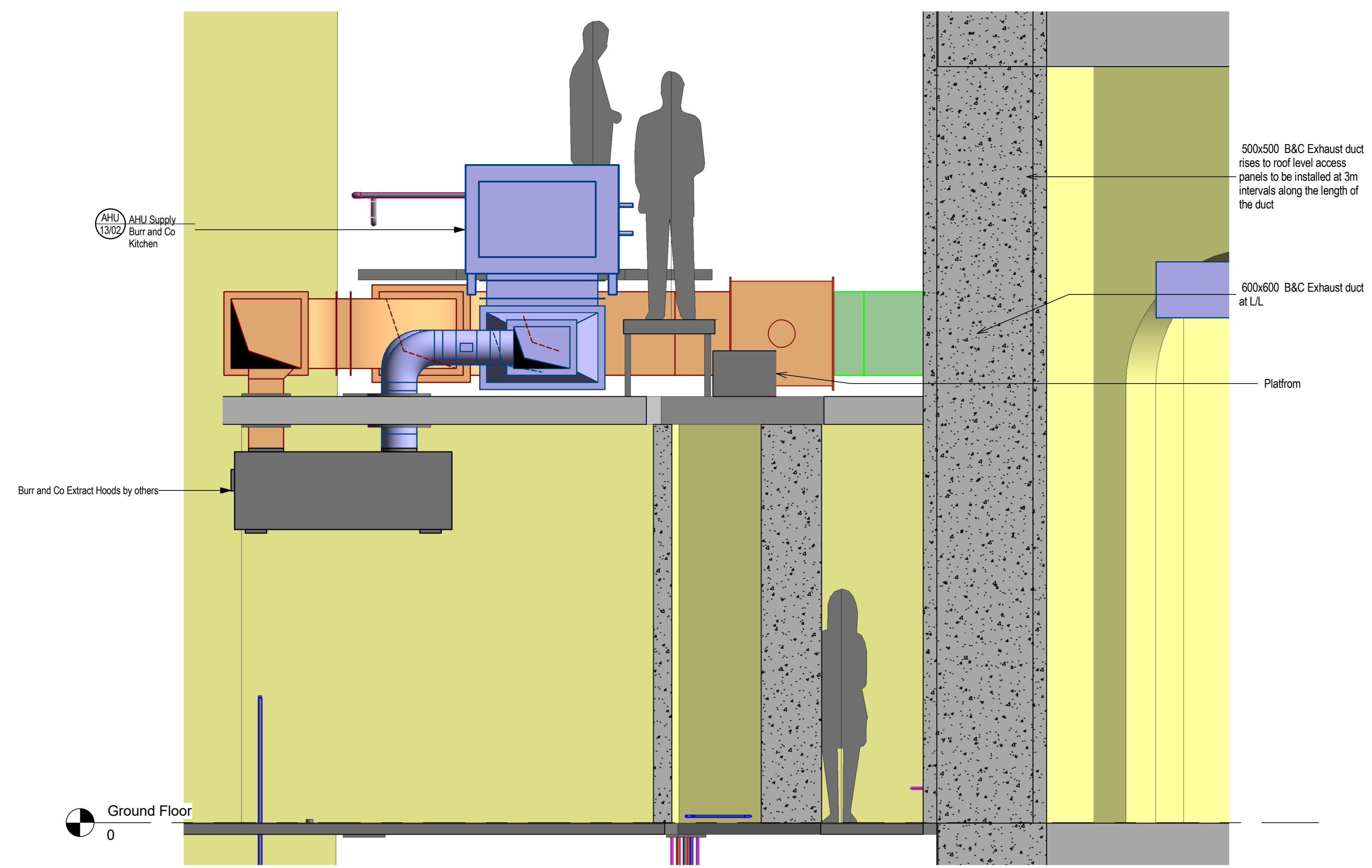
3 Section B - B 1 : 25
