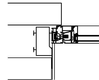
Jamb Detail Scale 1:10
