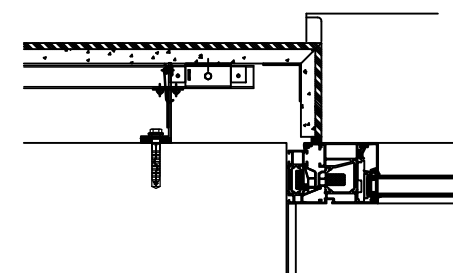
Jamb Detail Scale 1:10
