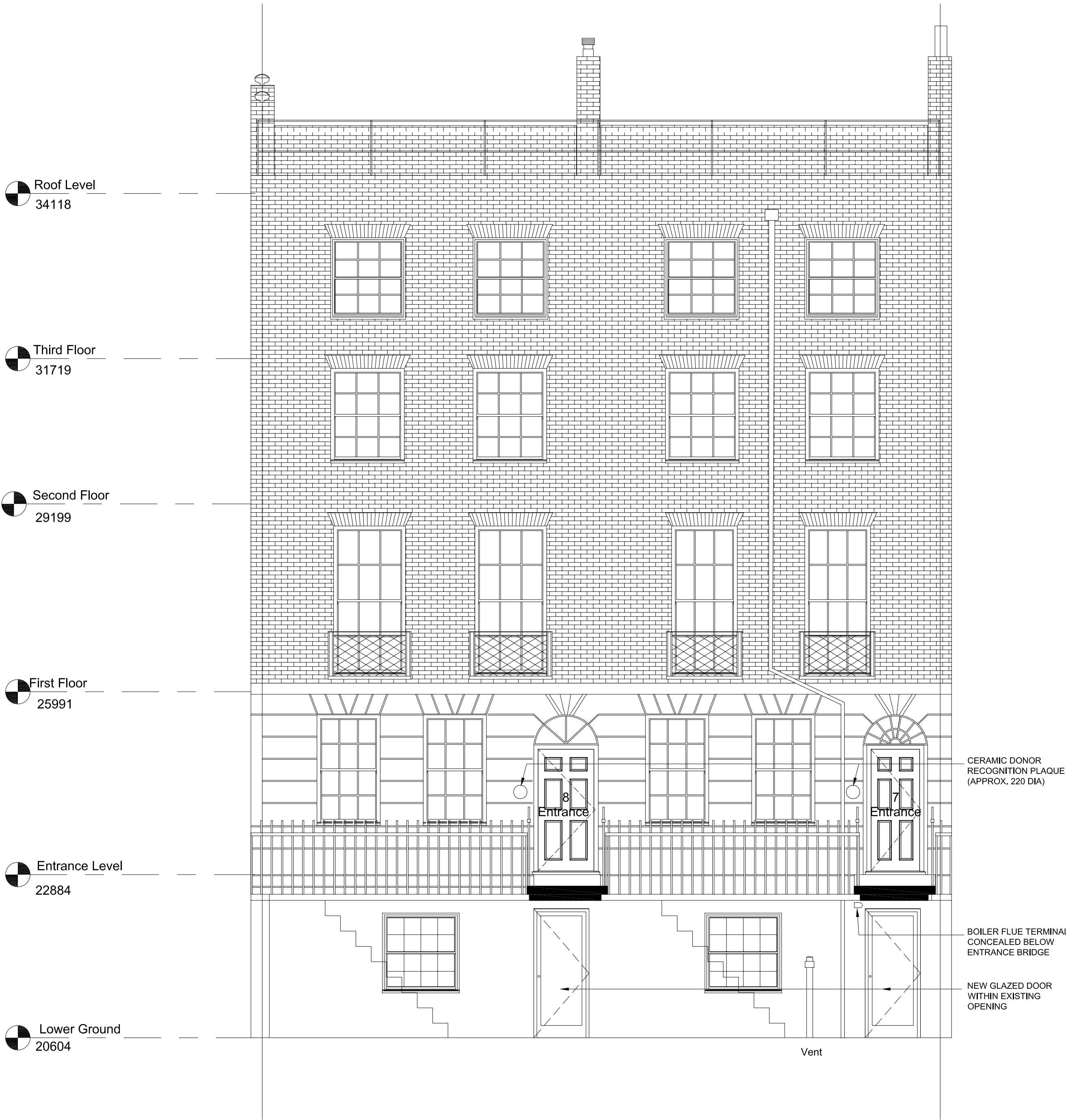
ELEVATION A
