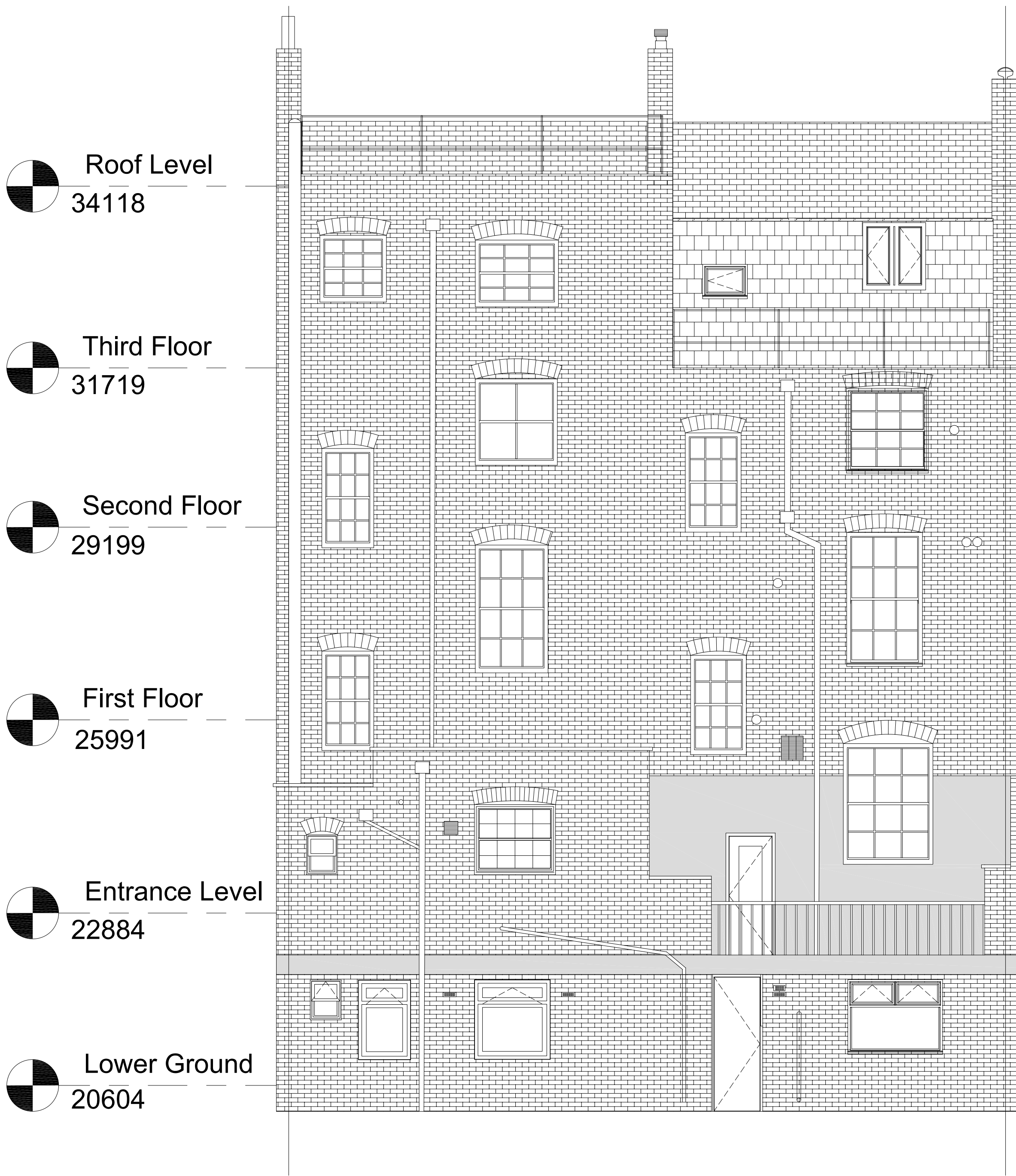
ELEVATION B
