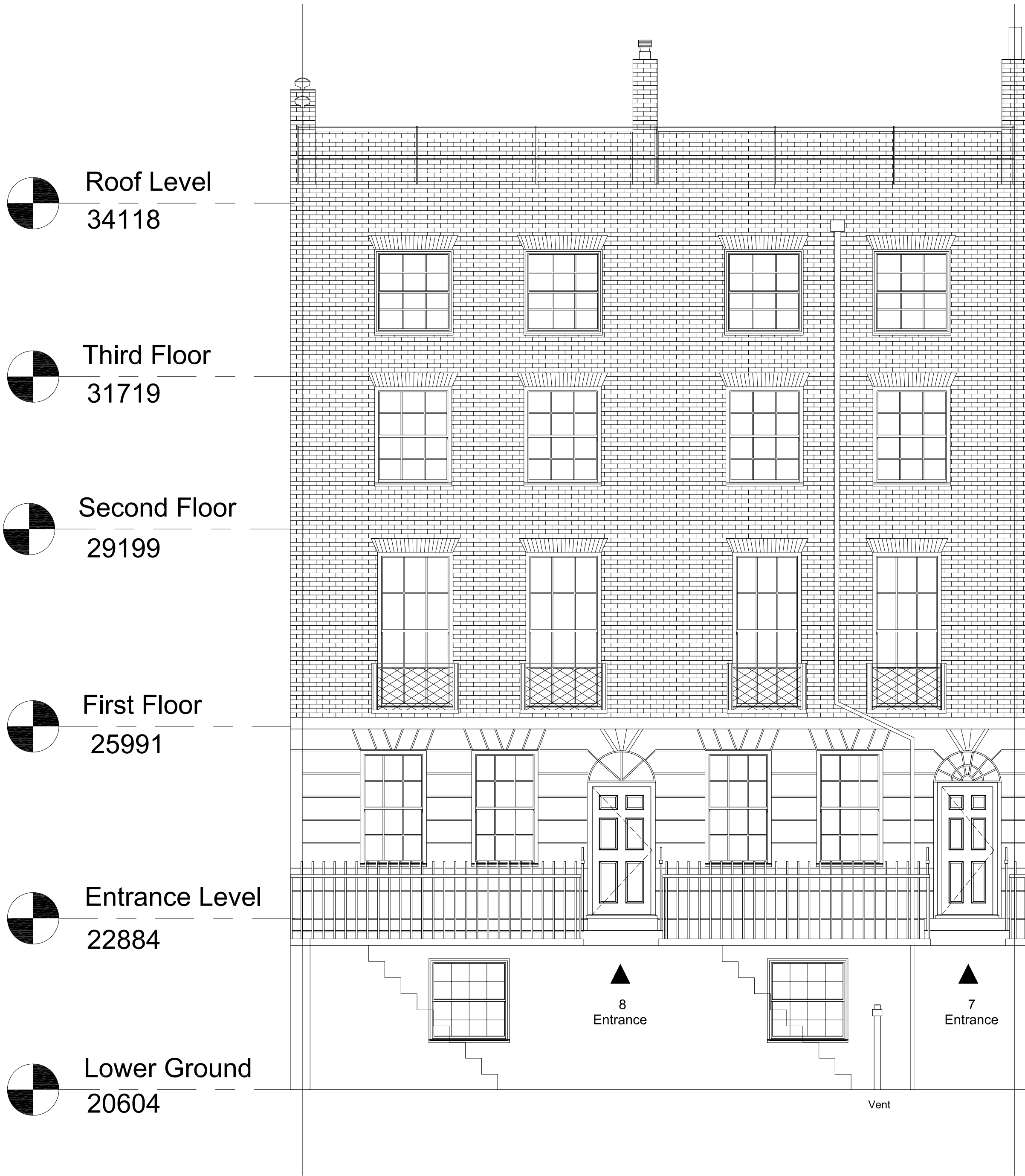
ELEVATION A
