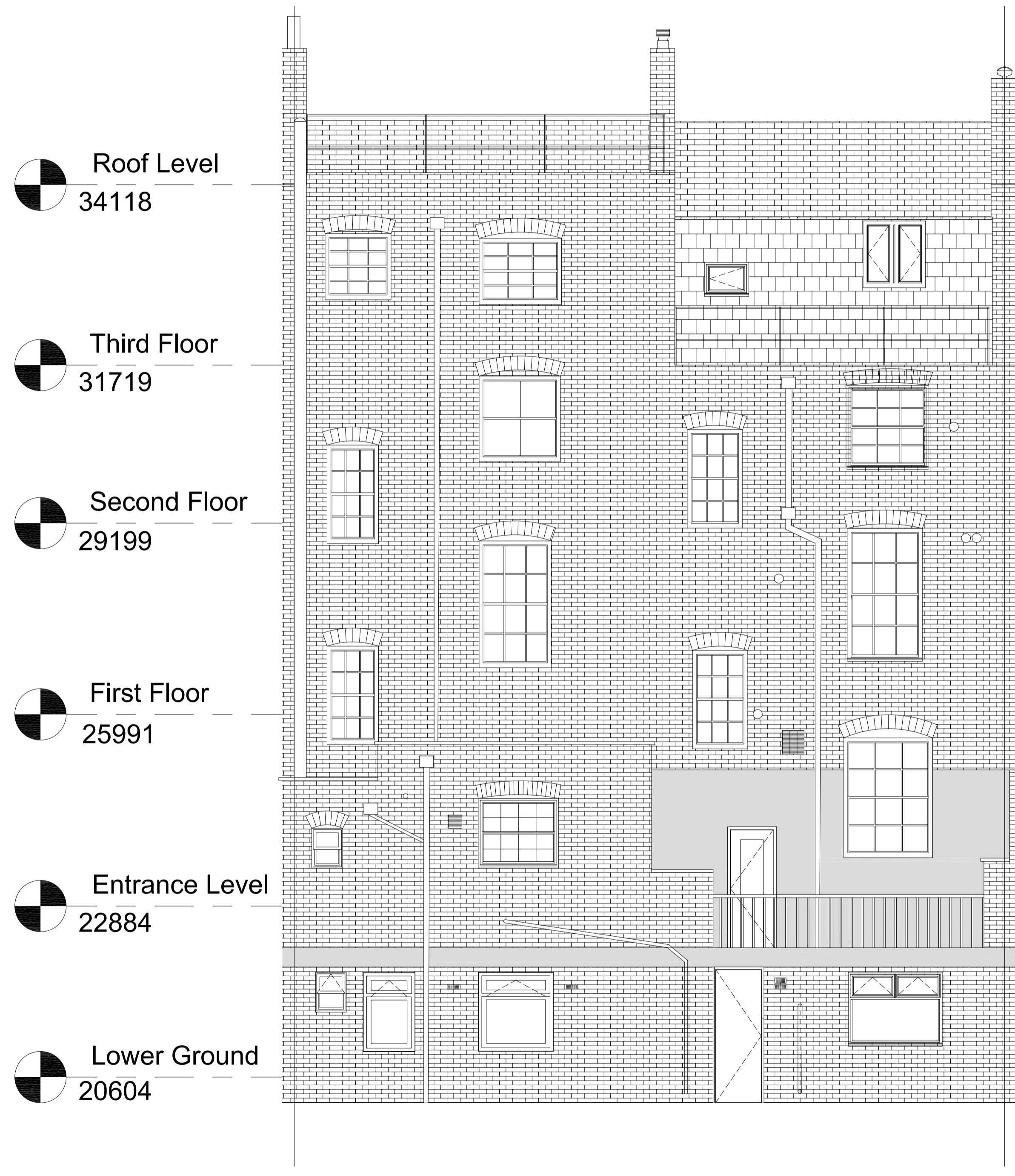
ELEVATION B
