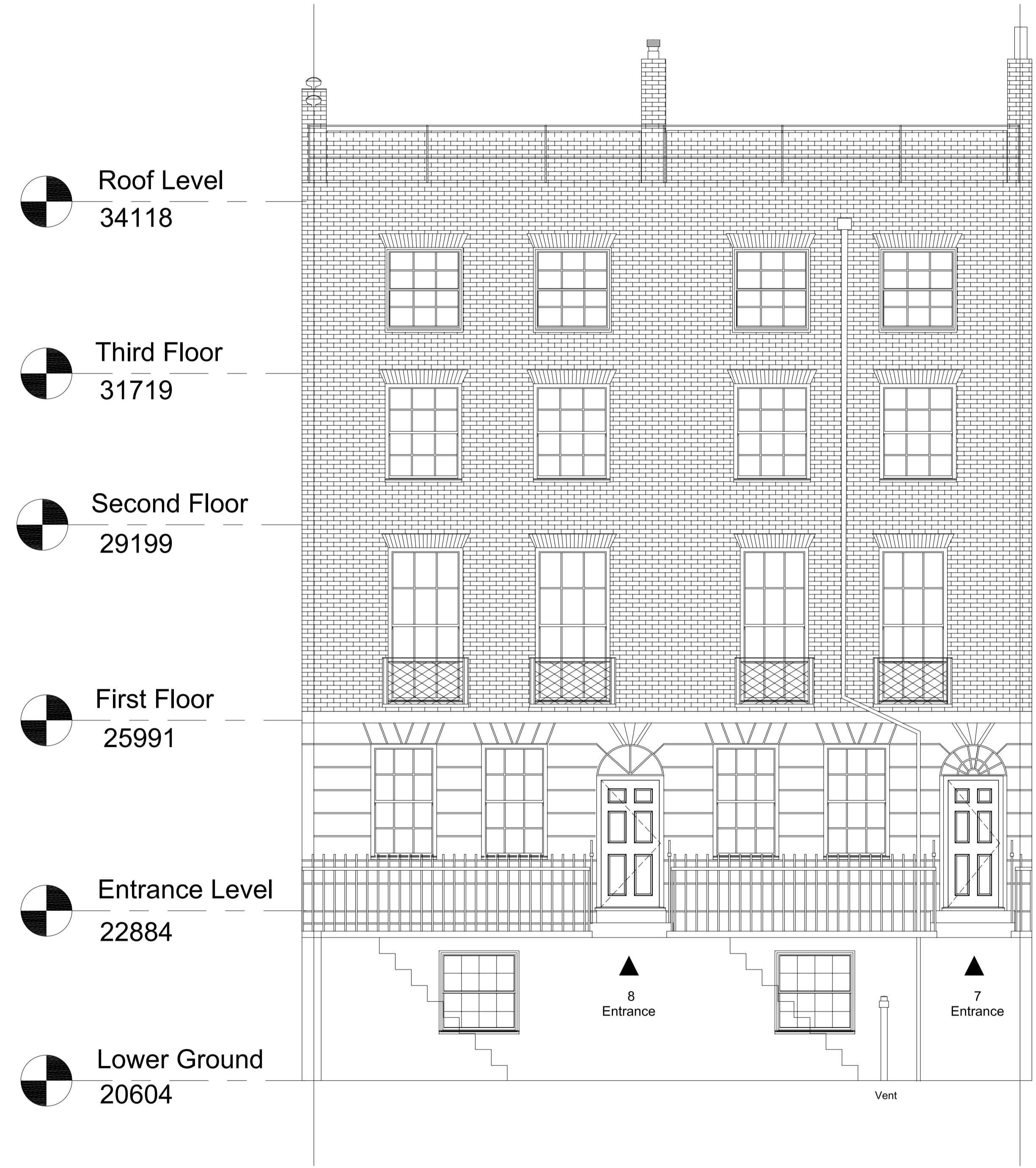
ELEVATION A
