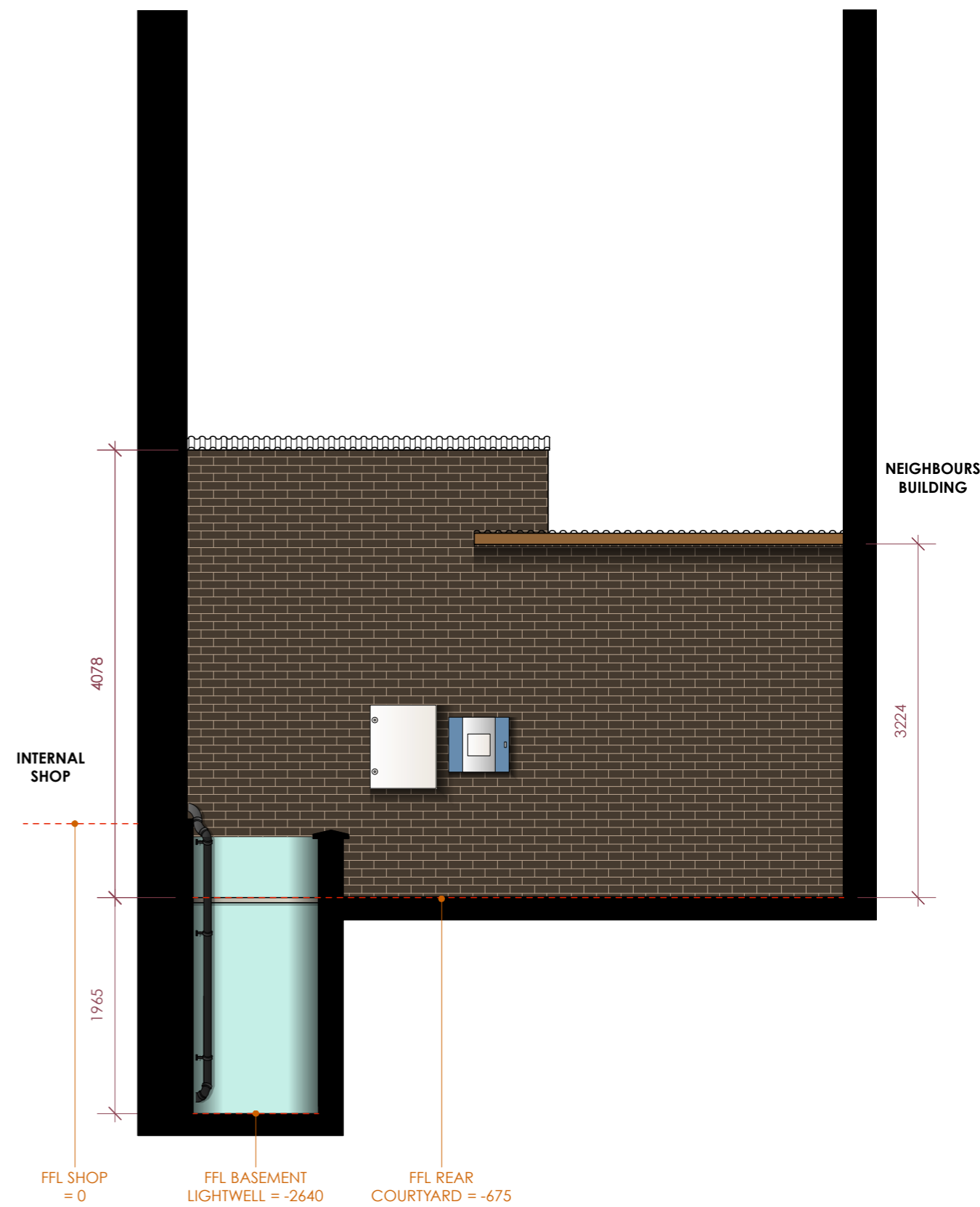
existing SECTION DD
