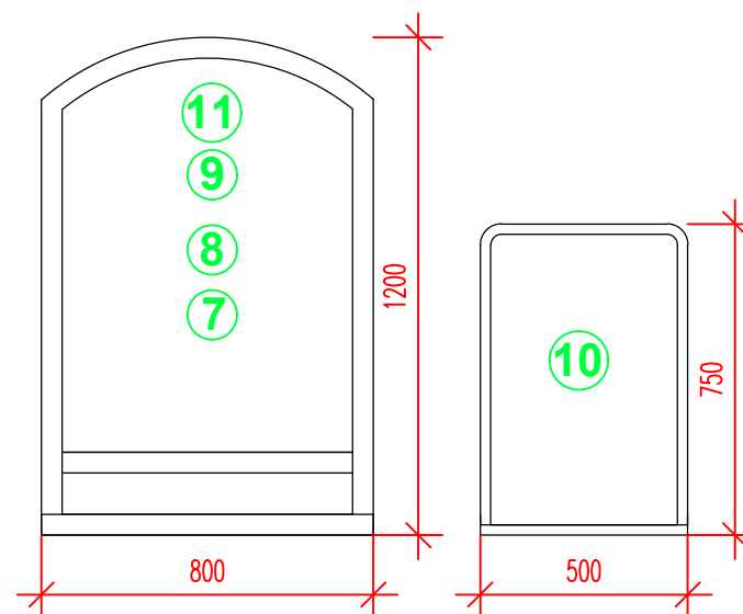
Scale 1:20 @ A3
