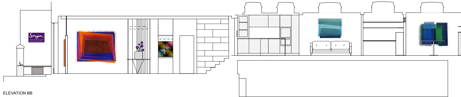
ELEVATION BB
