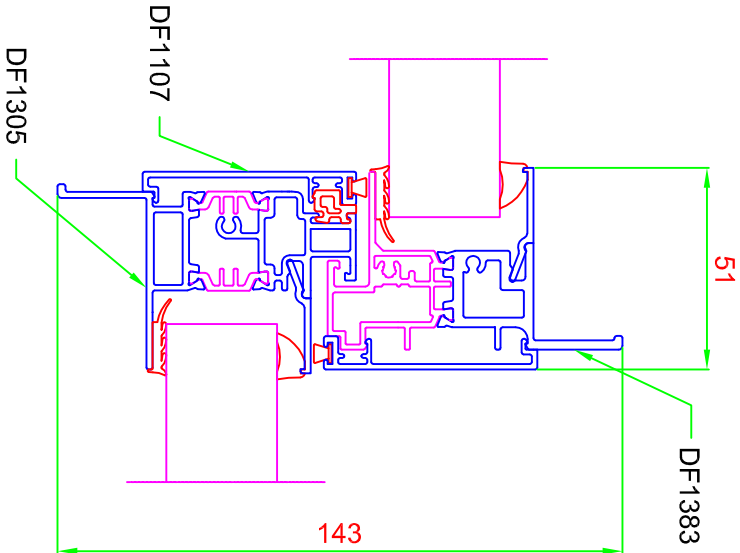
Section DD
