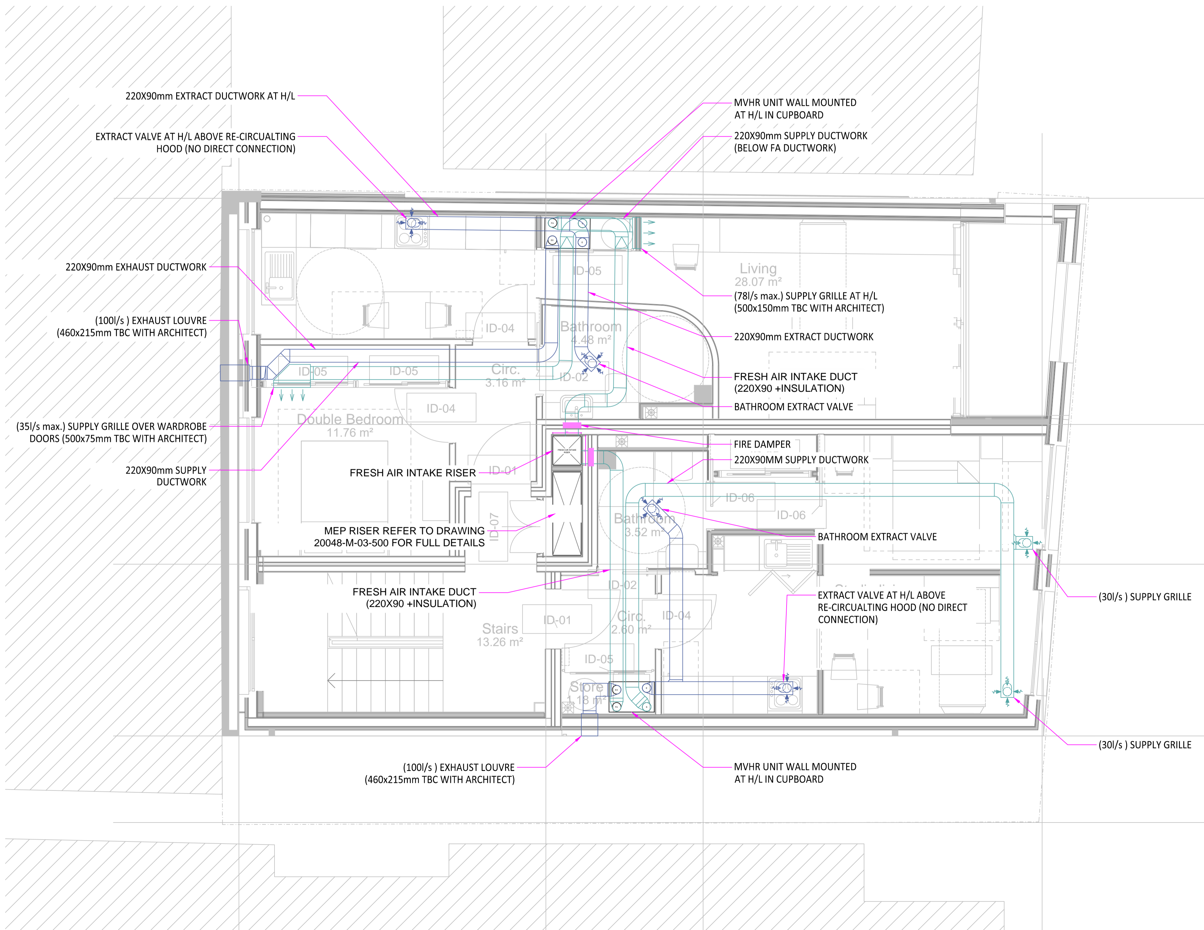
SC VENTILATION SCHEMATIC N.T.S
