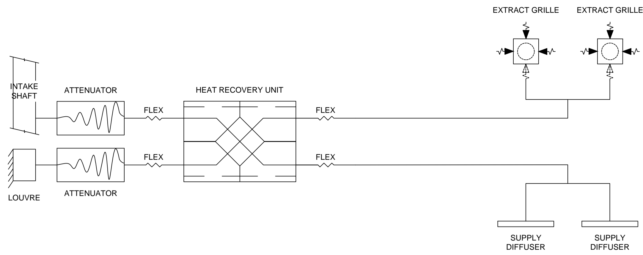
SC VENTILATION SCHEMATIC N.T.S
