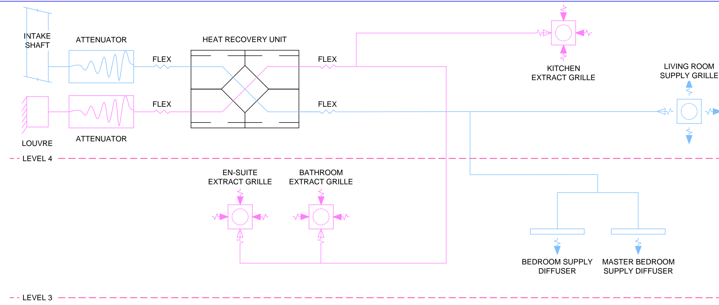
SC VENTILATION SCHEMATIC N.T.S
