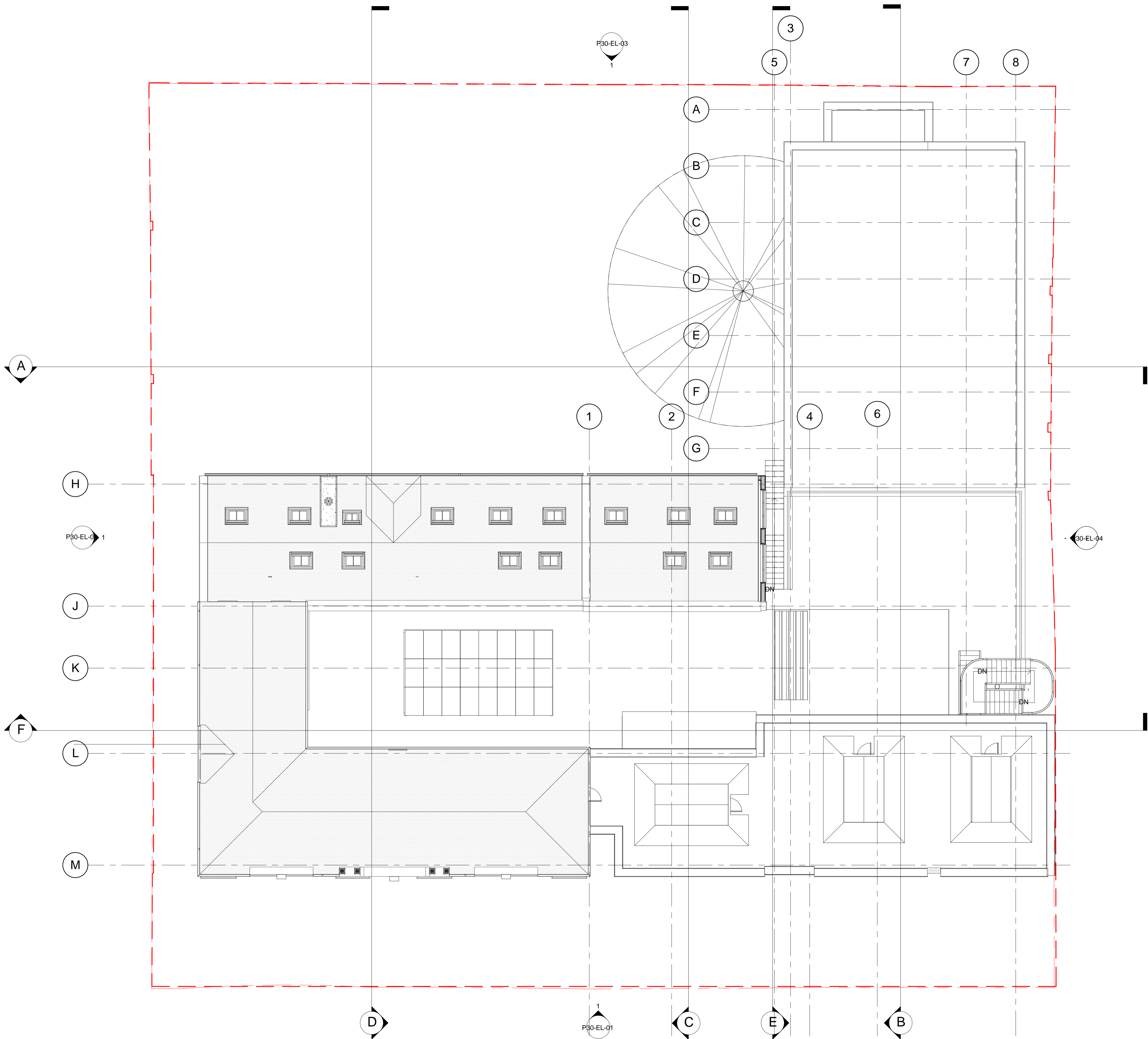
Existing L03 Roof 1 : 100
