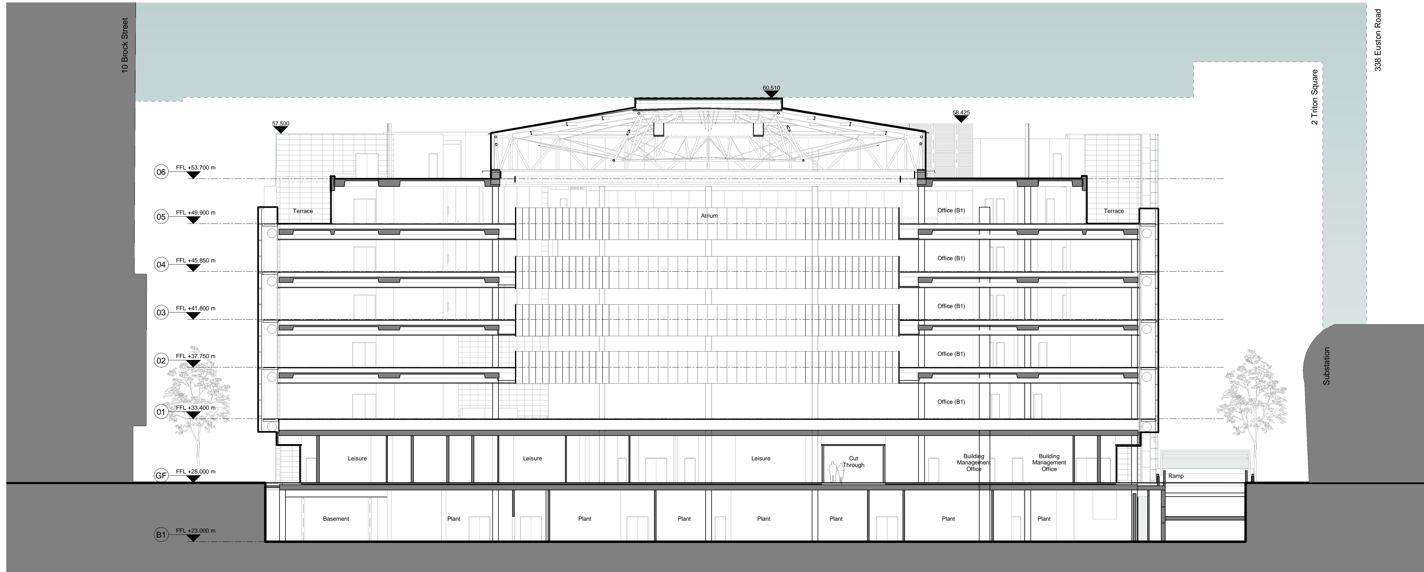
2 Section BB 1 : 200
