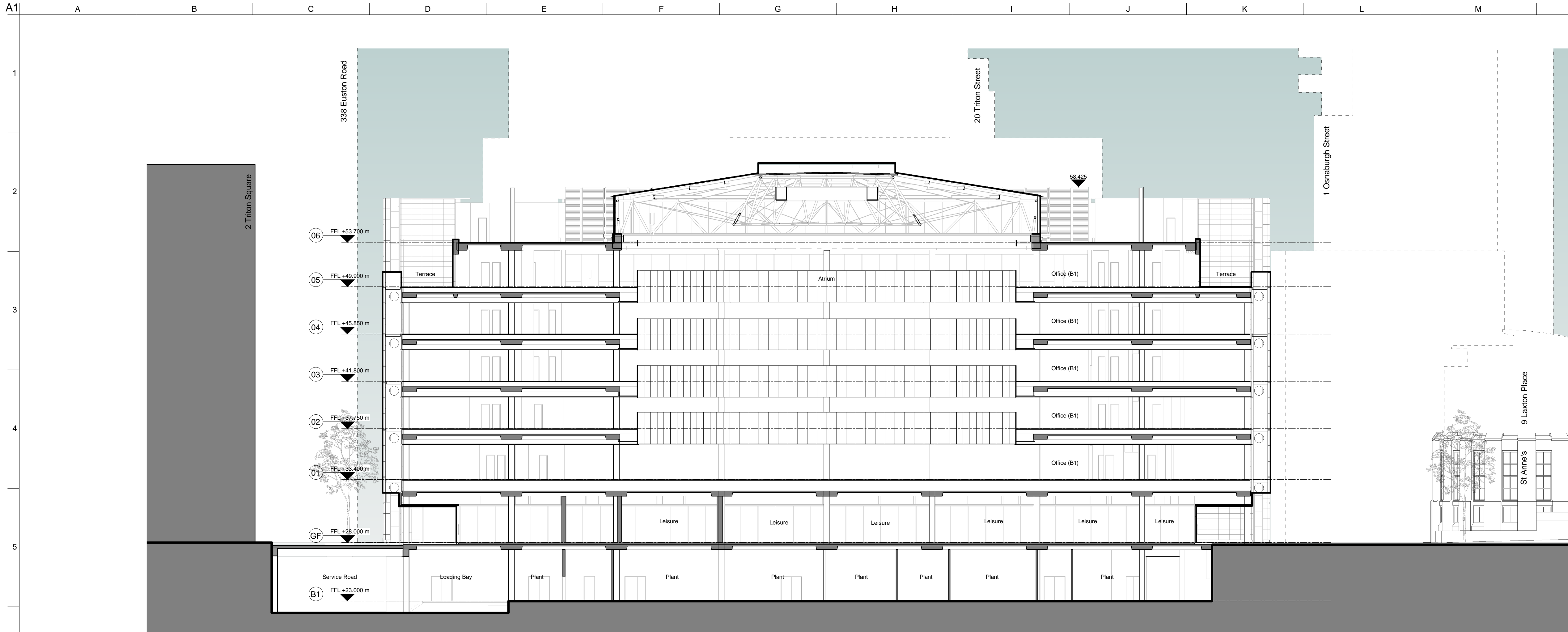
1 Section AA 1 : 200
