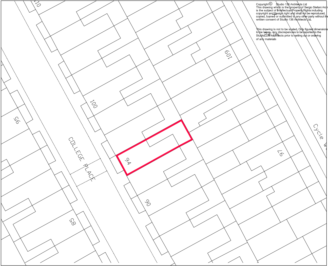
Site Plan 1:500
