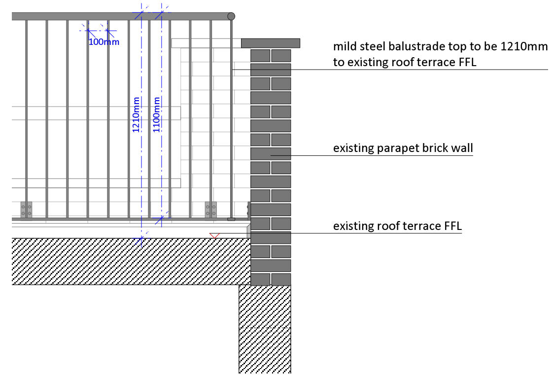
Detail section D'01 1:20
