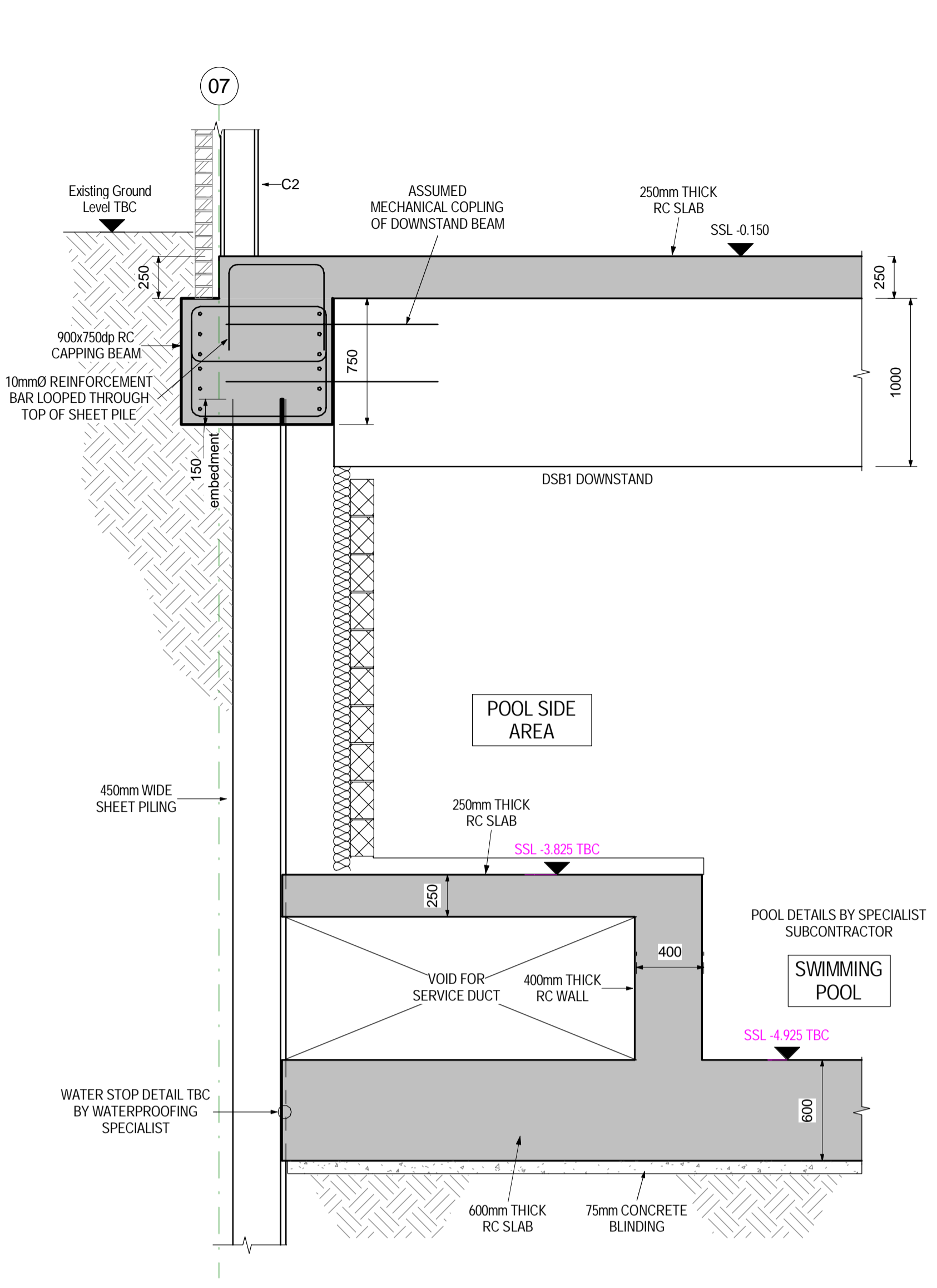
03 SECTION 1 : 25
