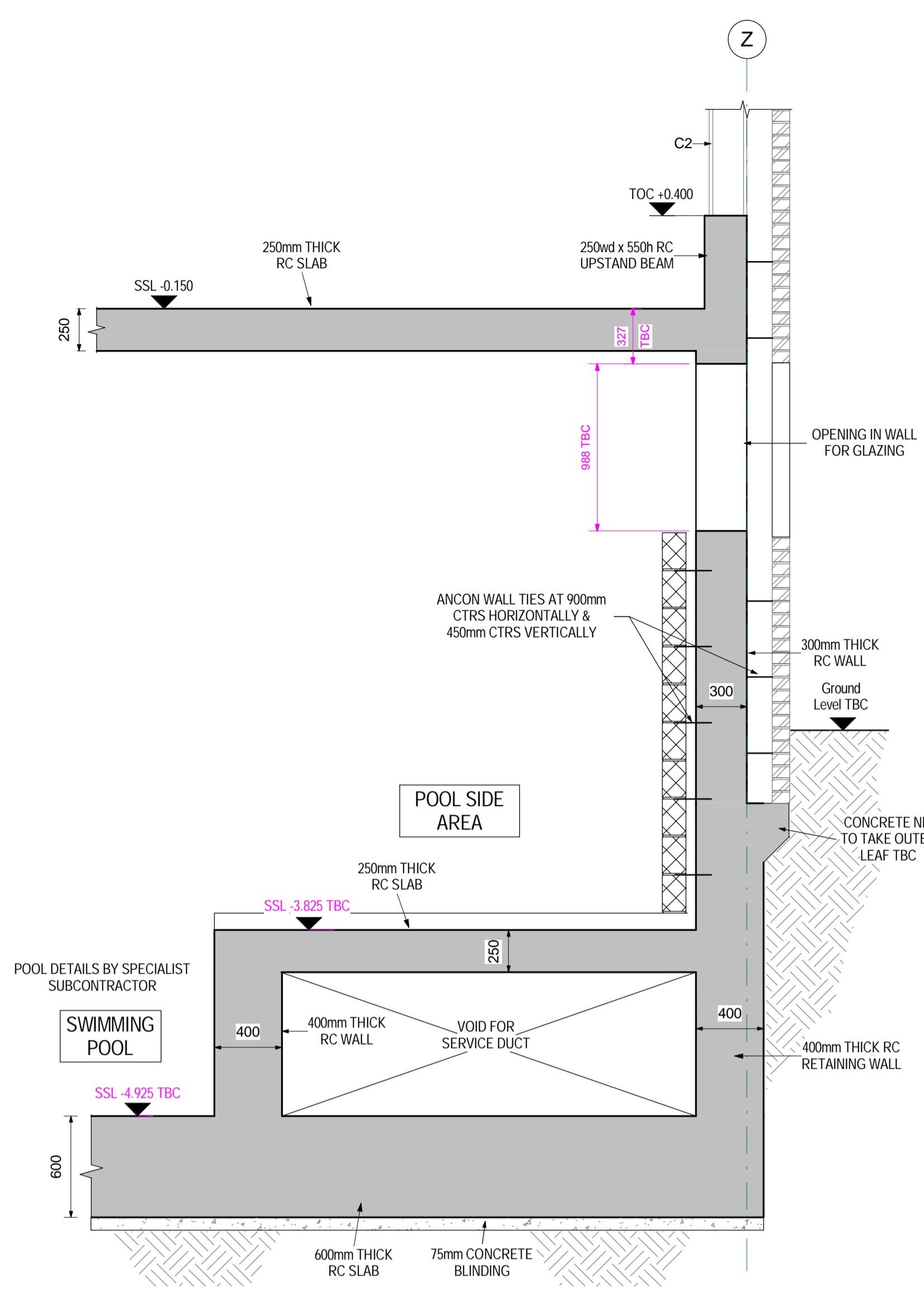
02 SECTION 1 : 25
