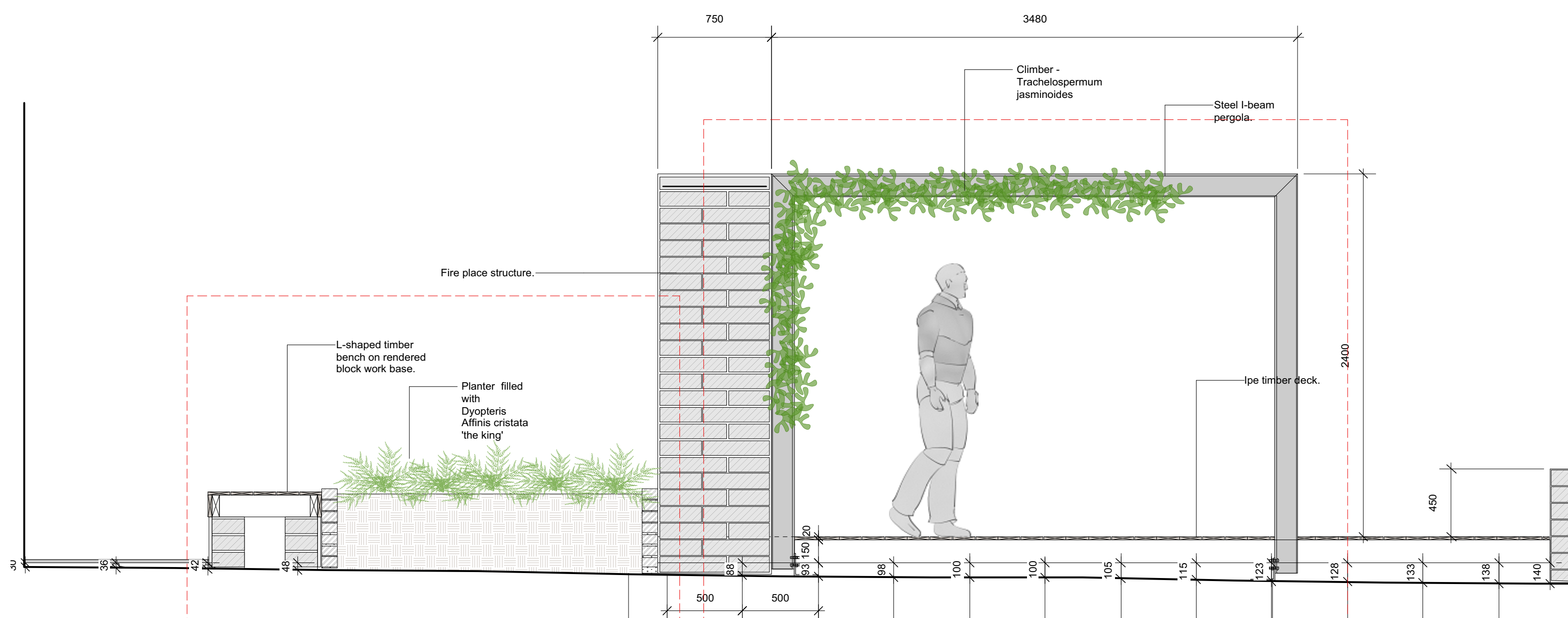
Basement roof membrane 2 Section A-A Scale: 1:25
