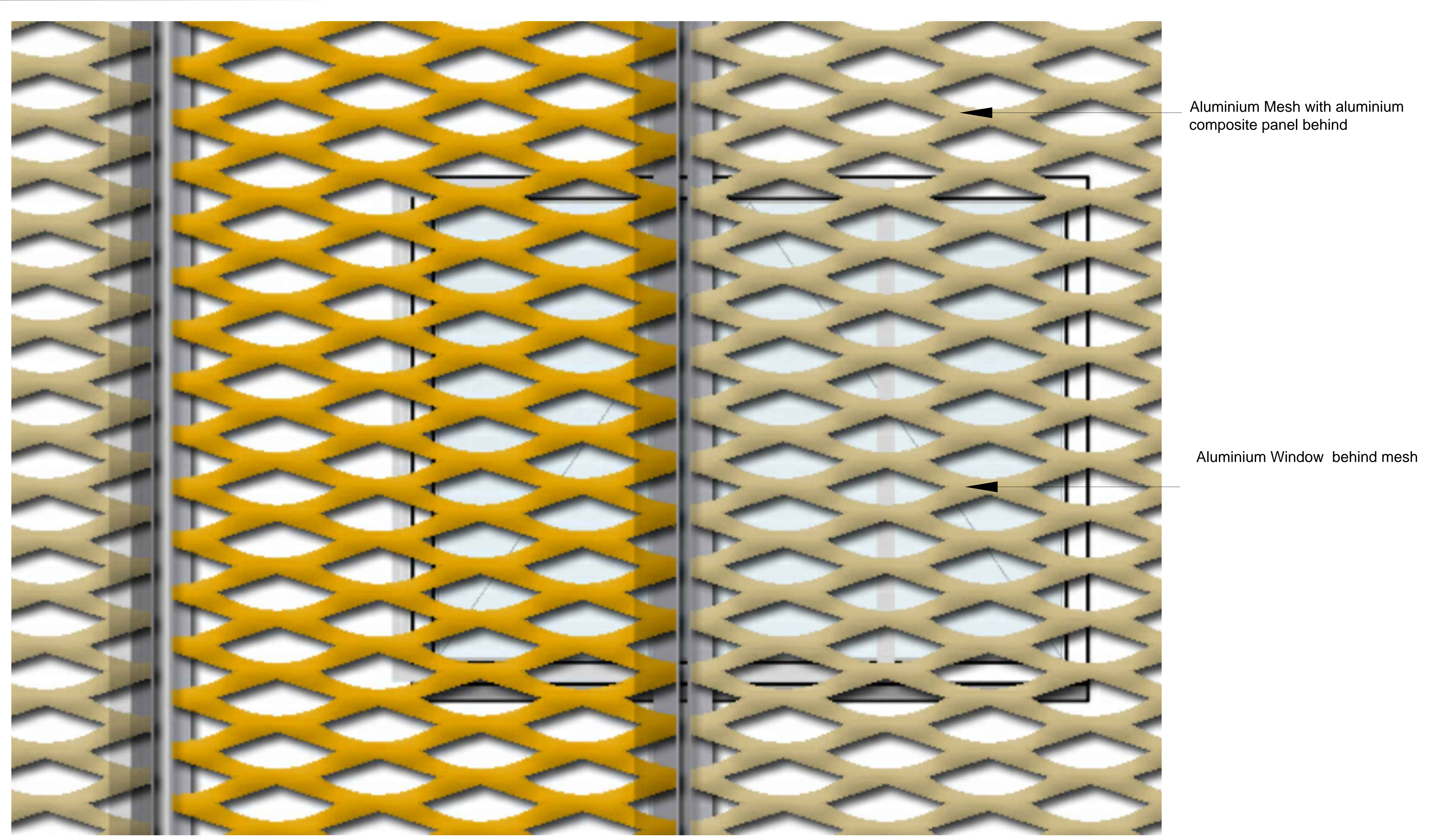
PARTIAL ELEVATION S. 1:5
