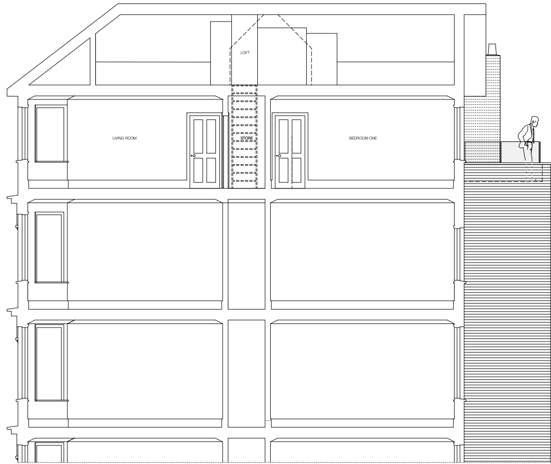
SECTION A-A
