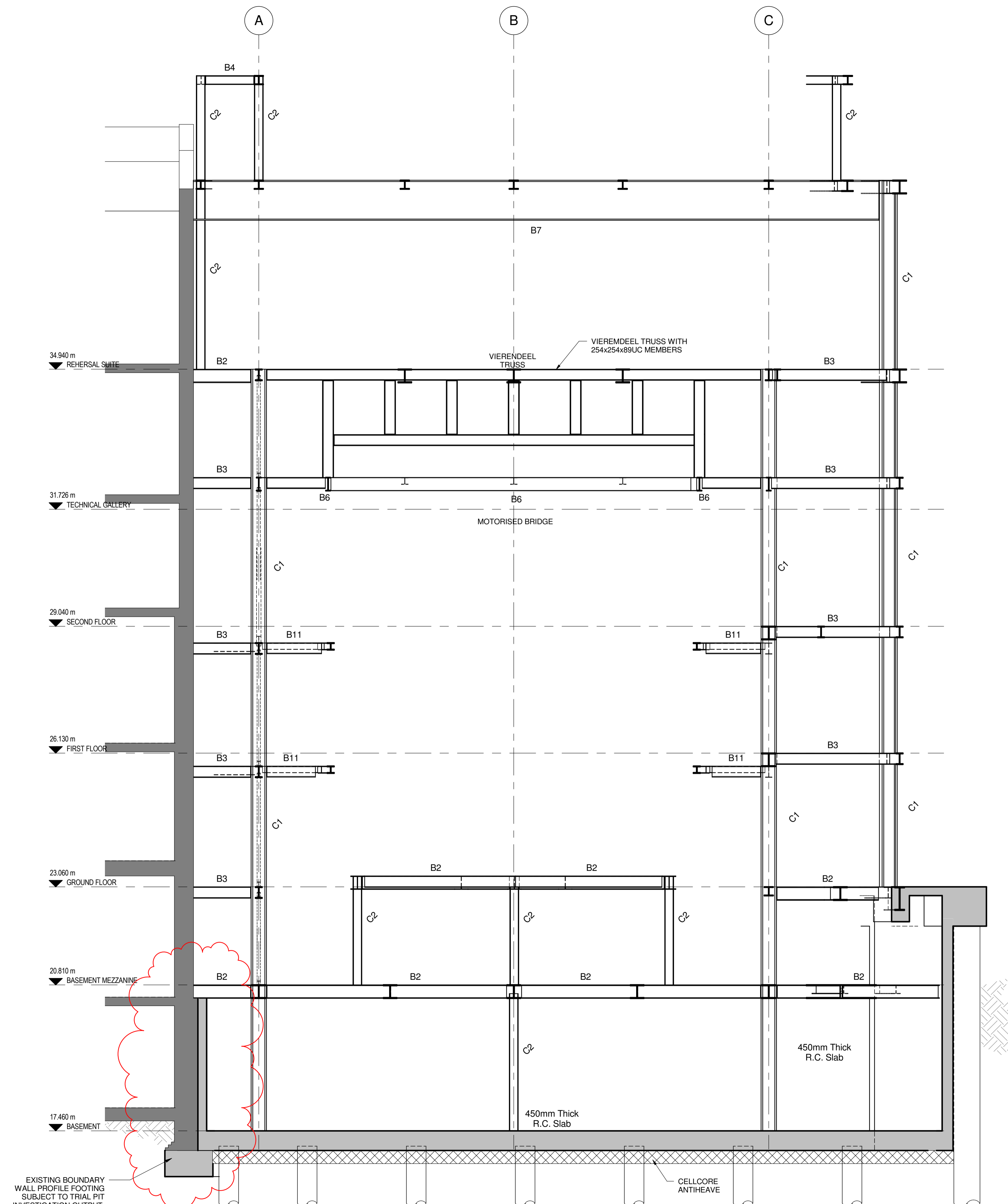
B Section B-B 1 : 50
