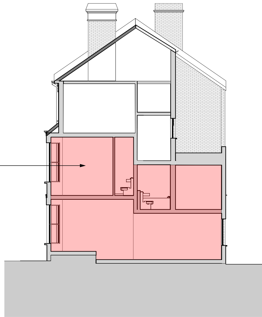
Section A2
