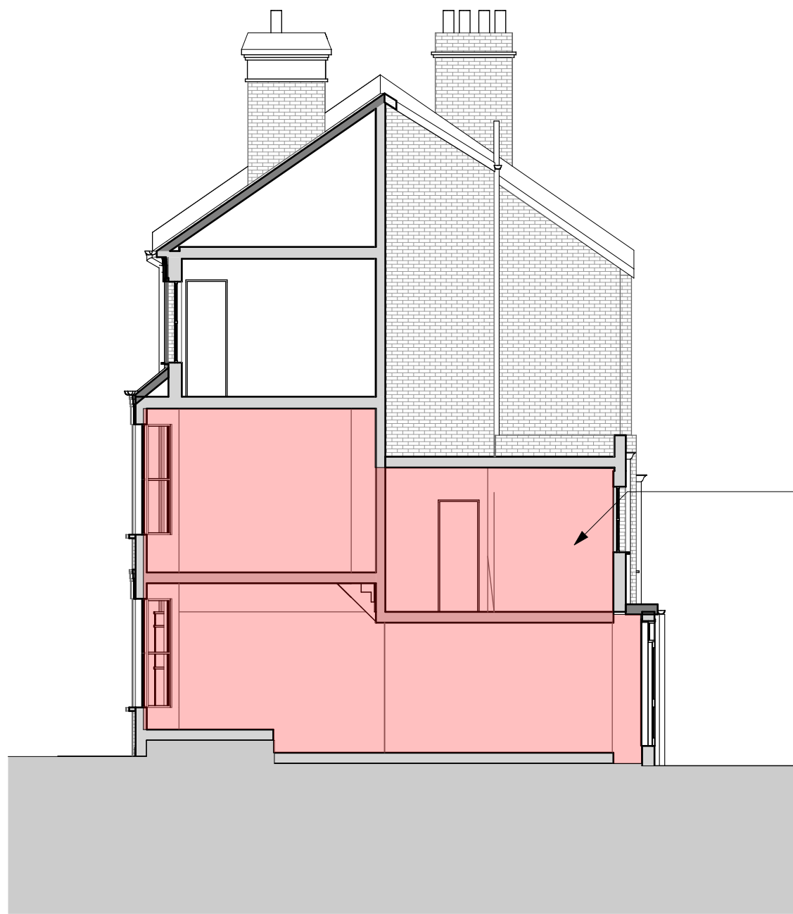
Section A1
