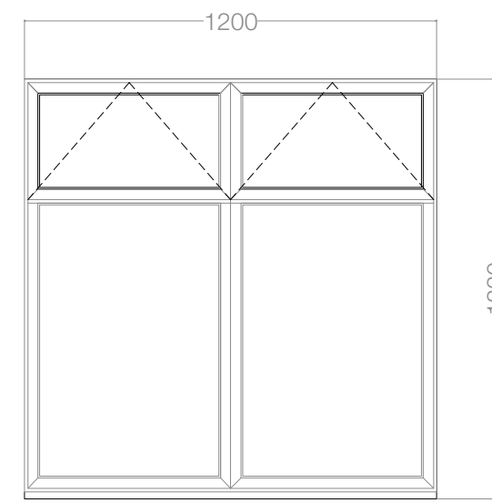
EW10 1:20 @ A1
