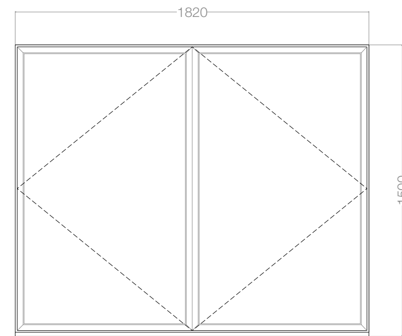
EW15 1:20 @ A1
