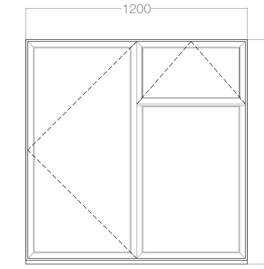
EW6 1:20 @ A1
