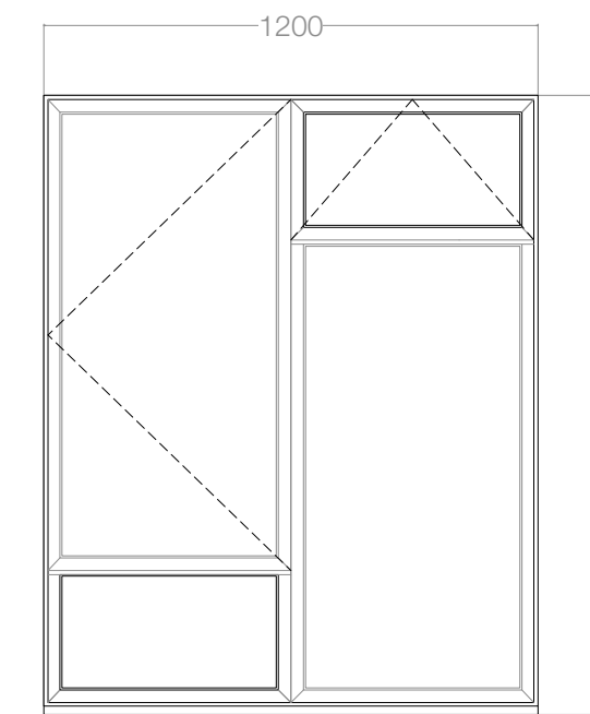
EW18 1:20 @ A1
