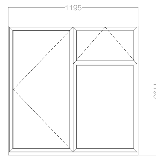
EW1 1:20 @ A1
