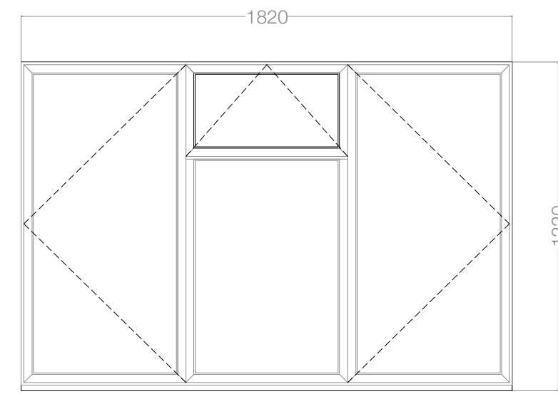
EW9 1:20 @ A1
