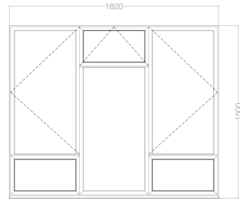
EW8 1:20 @ A1
