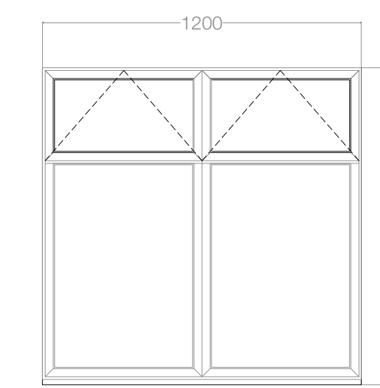
EW11 1:20 @ A1
