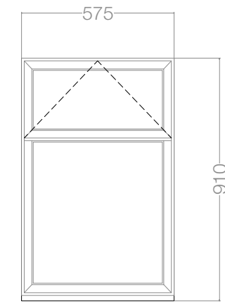
EW2 1:20 @ A1
