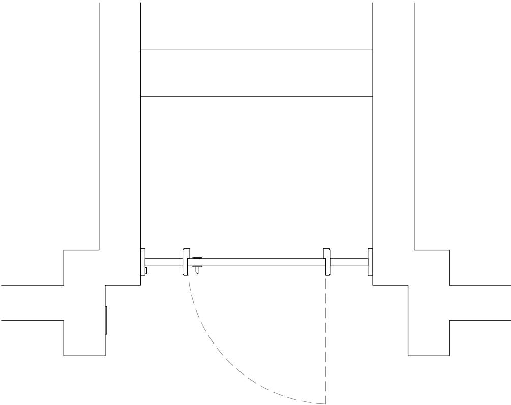
02 A300 PLAN DOOR 21_110-117 SCALE 1:25
