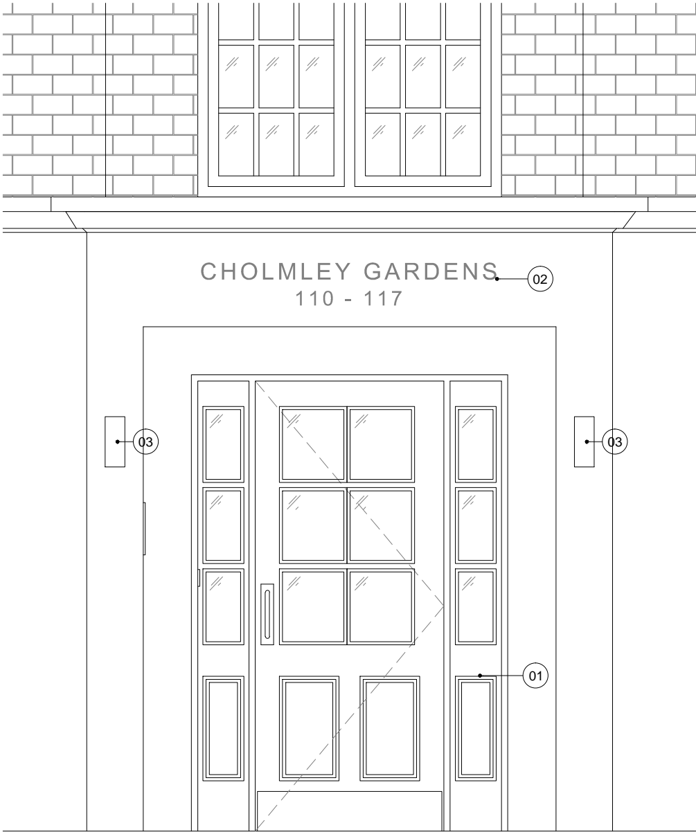
01 A300 ELEVATION DOOR 21_110-117 SCALE 1:25
