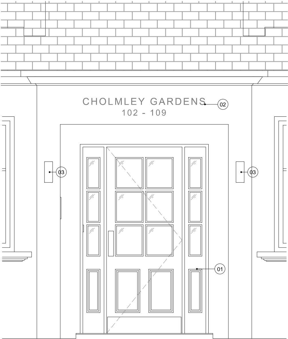
01 A290 ELEVATION DOOR 20_102-109 SCALE 1:25
