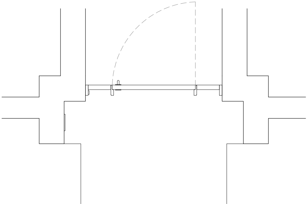
02 A290 PLAN DOOR 20_102-109 SCALE 1:25
