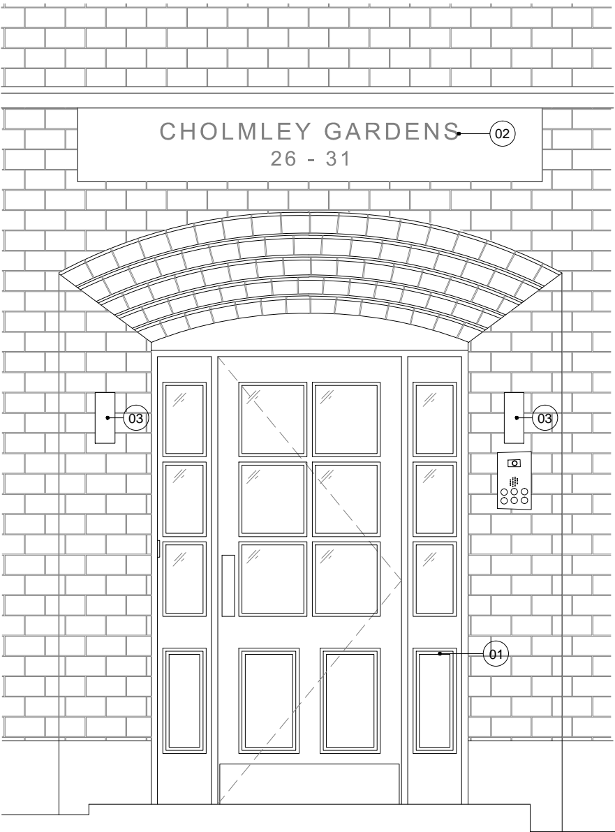
01 ELEVATION DOOR 9_26-31 A180 SCALE 1:25
