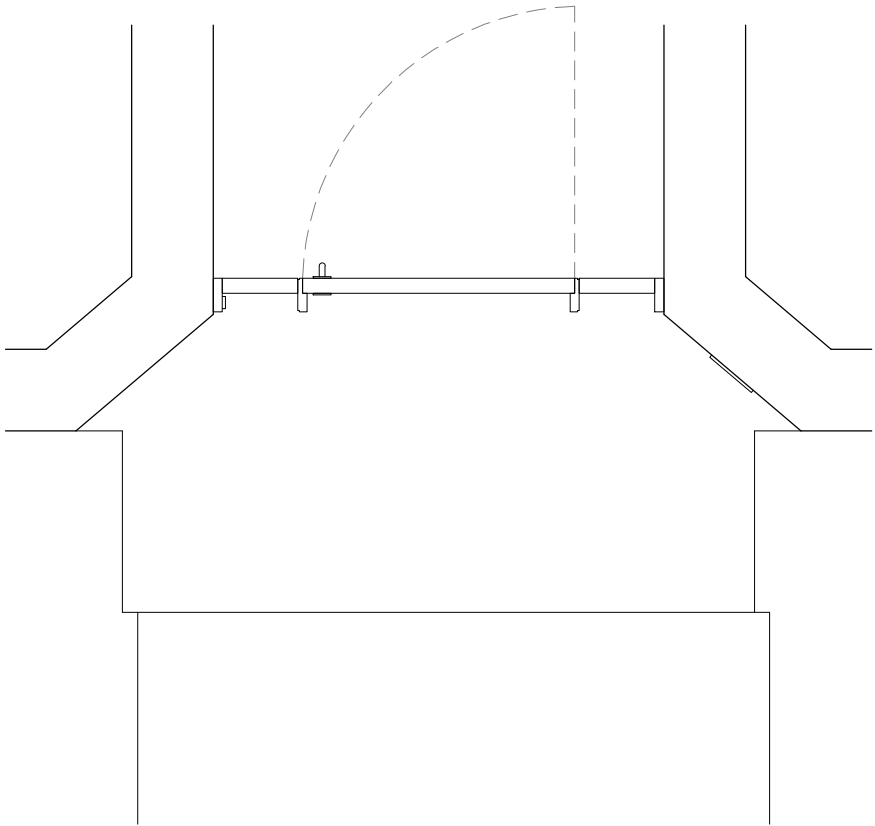
02 A160 PLAN DOOR 7_14-19 SCALE 1:25
