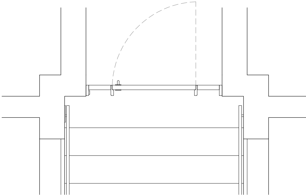
02 A120 PLAN DOOR 3_150-157 SCALE 1:25
