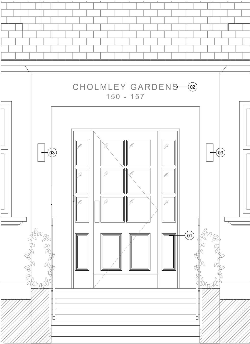
01 A120 ELEVATION DOOR 3_150-157 SCALE 1:25
