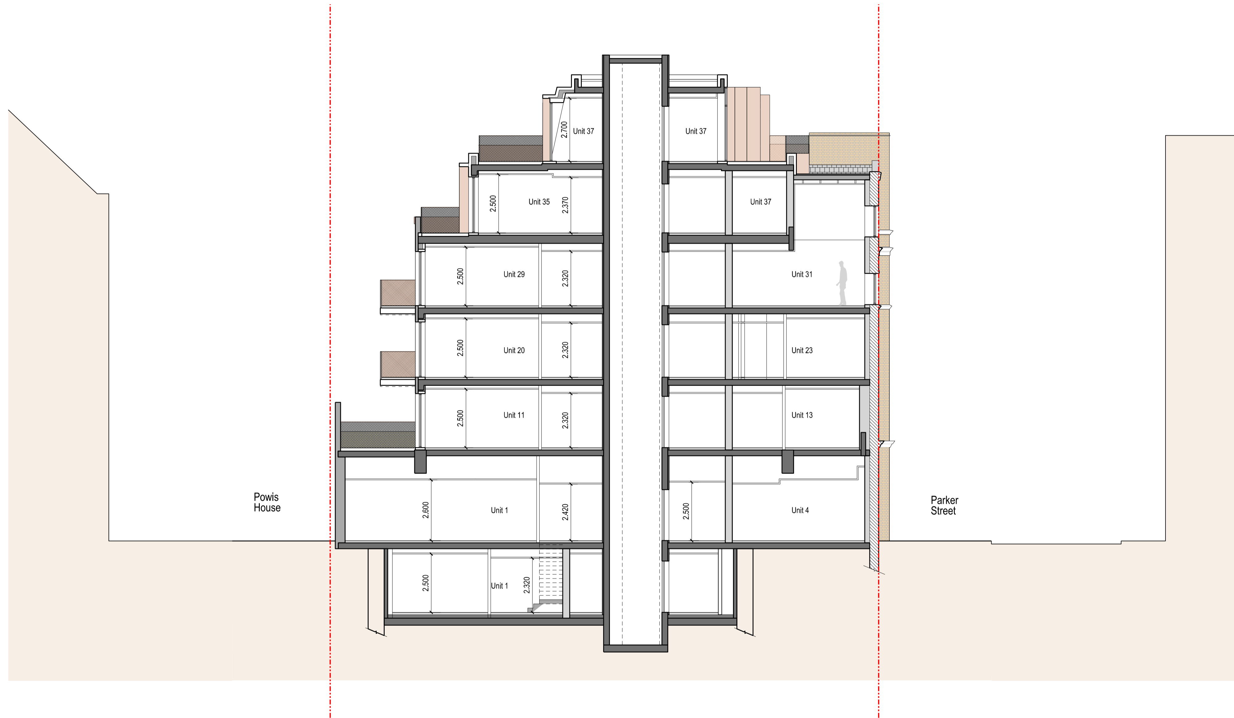
01 Section J-J 1:100
