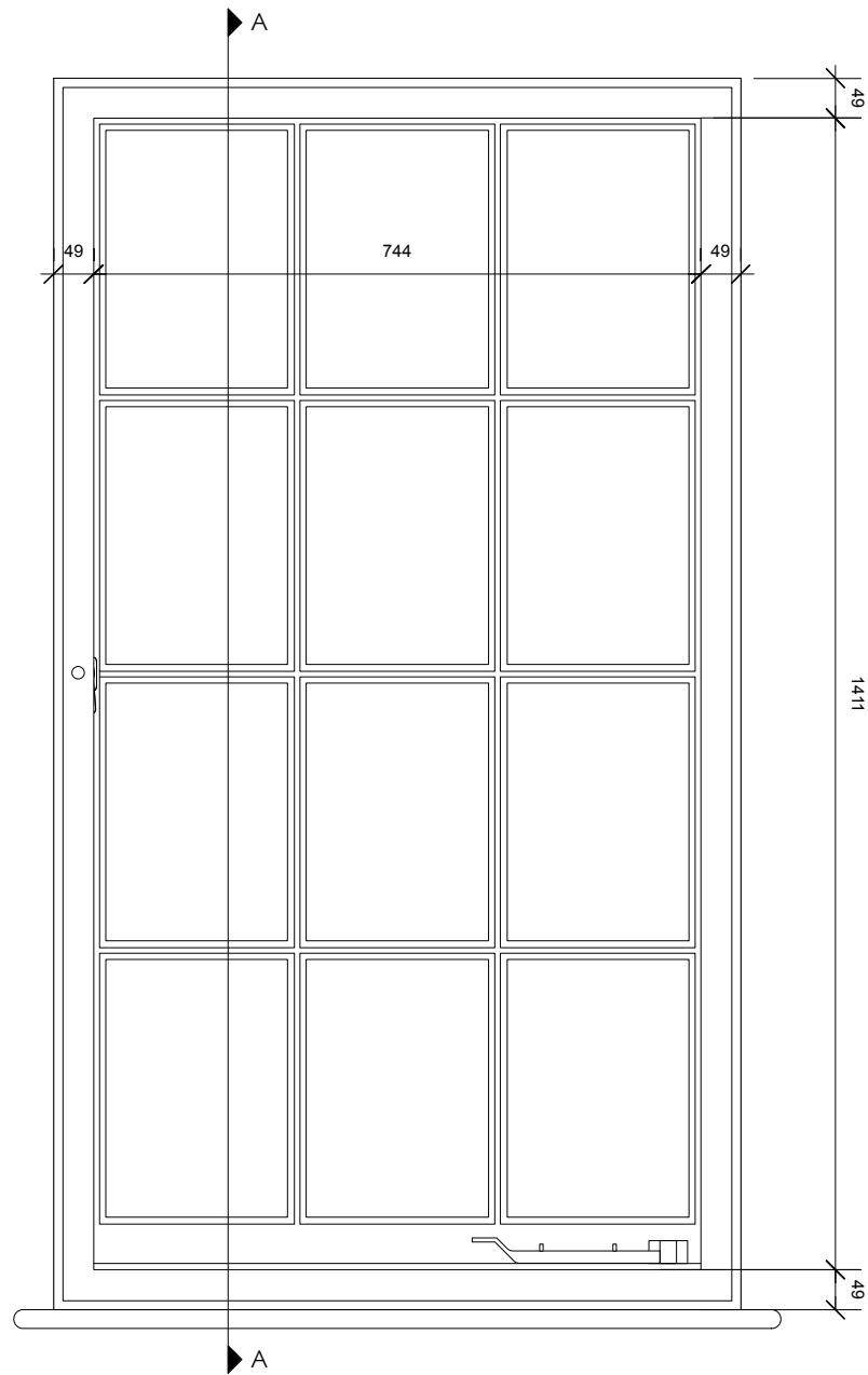
ELEVATION
