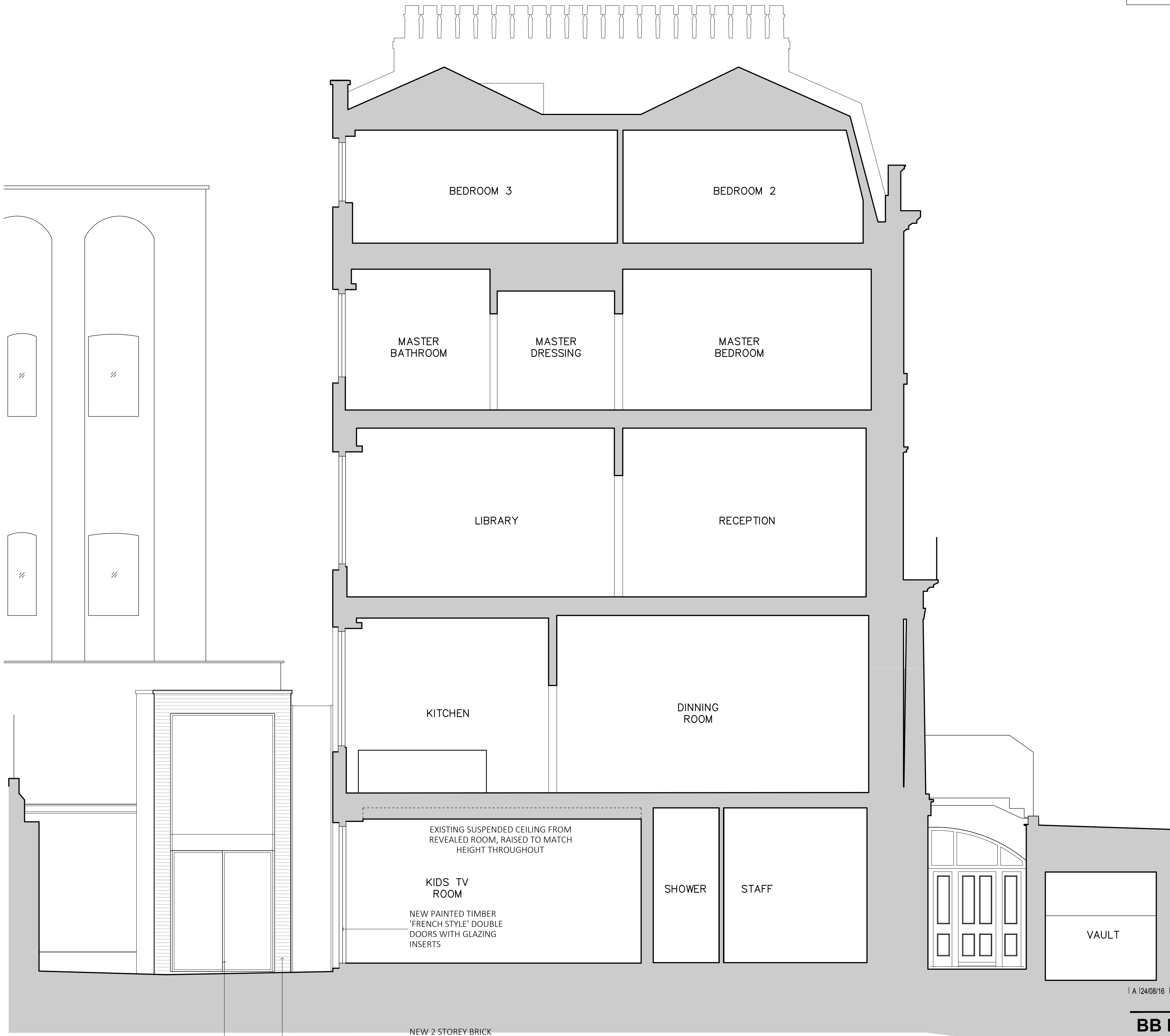
SECTION A-A
