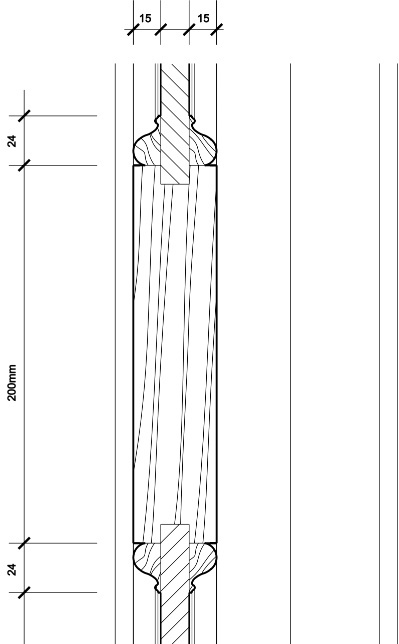
DOOR SECTION
