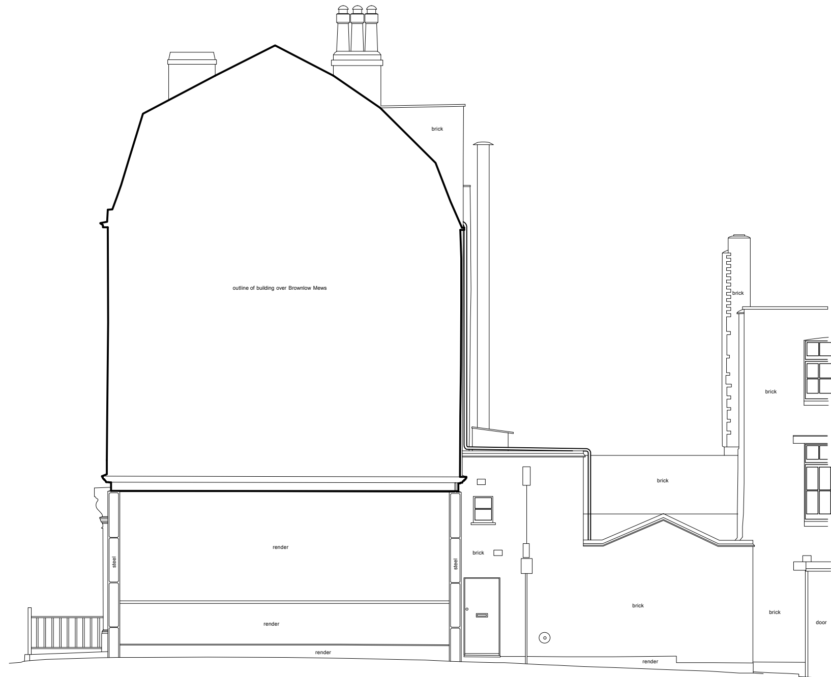
Flank Elevation
