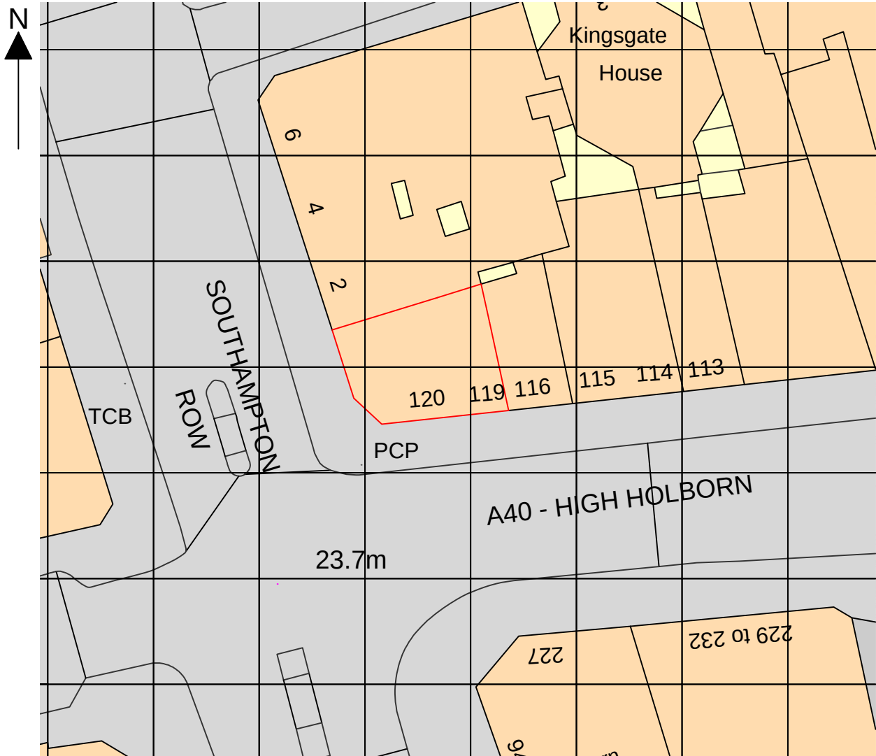
Site Plan 1:500
