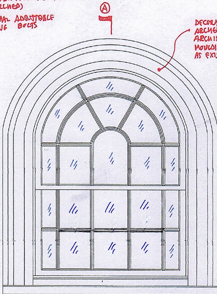
ELEVATION
