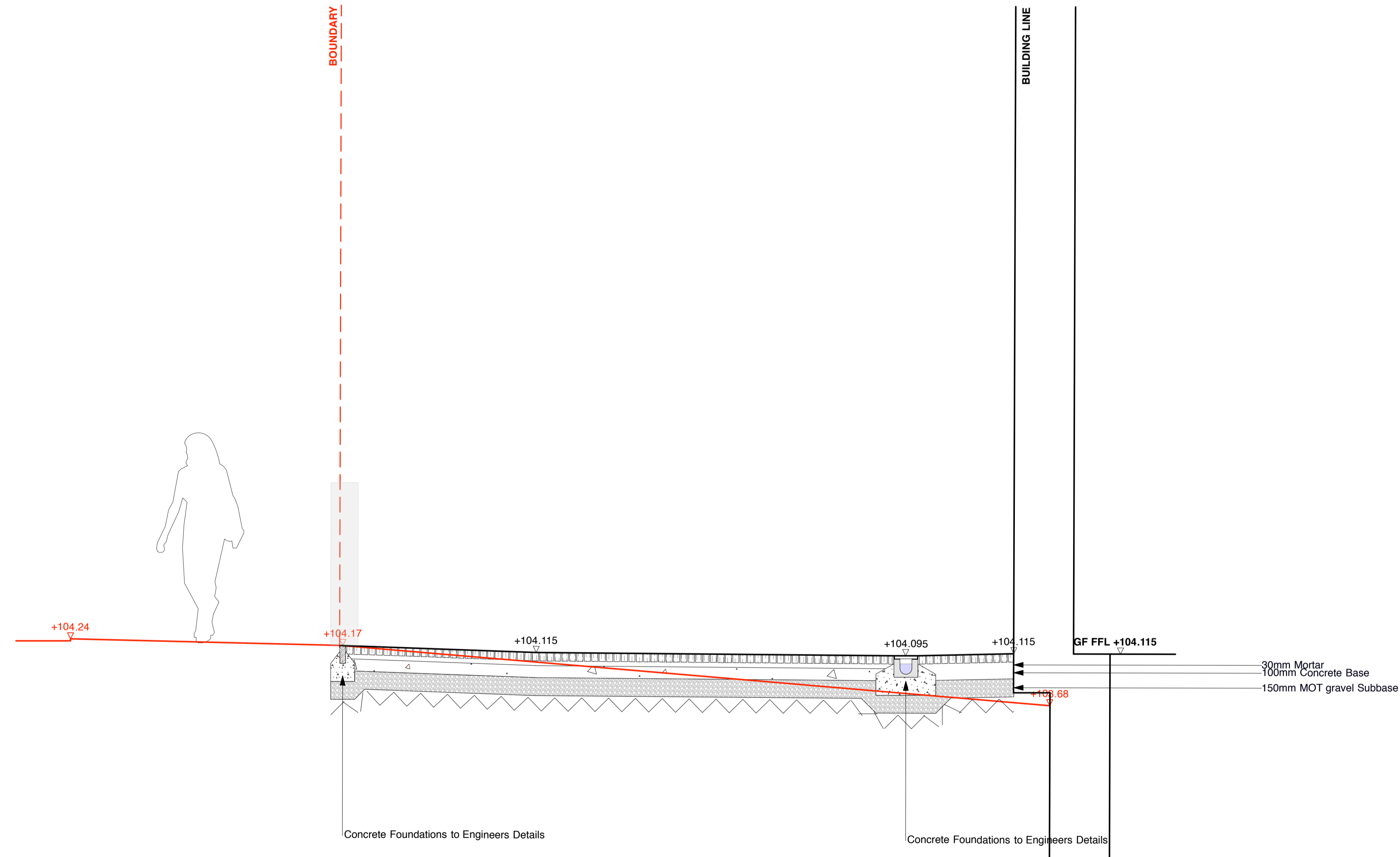
Section G - G' Scale: 1:25 at A1
