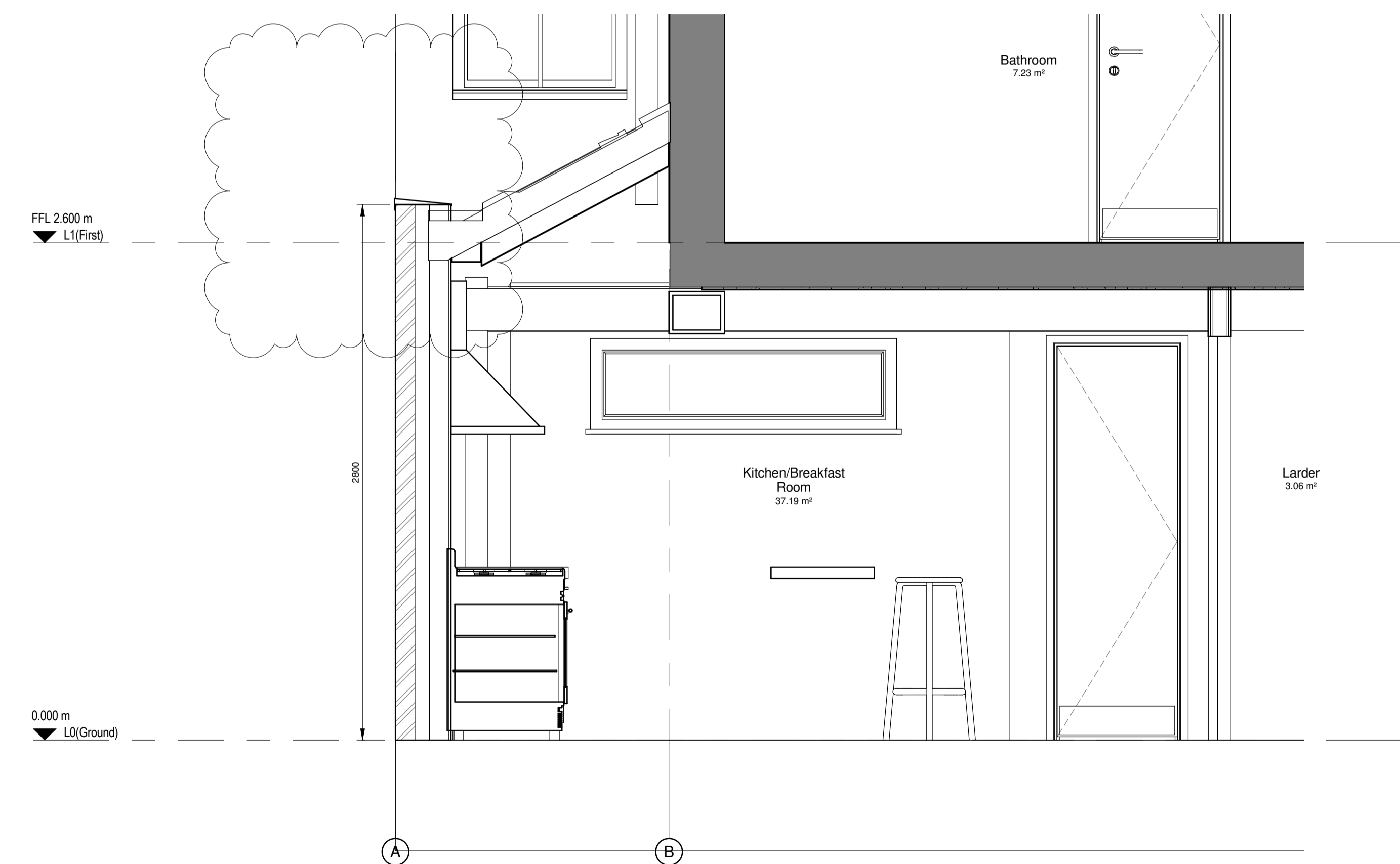
3.1 Elevation 3.1 1:20
