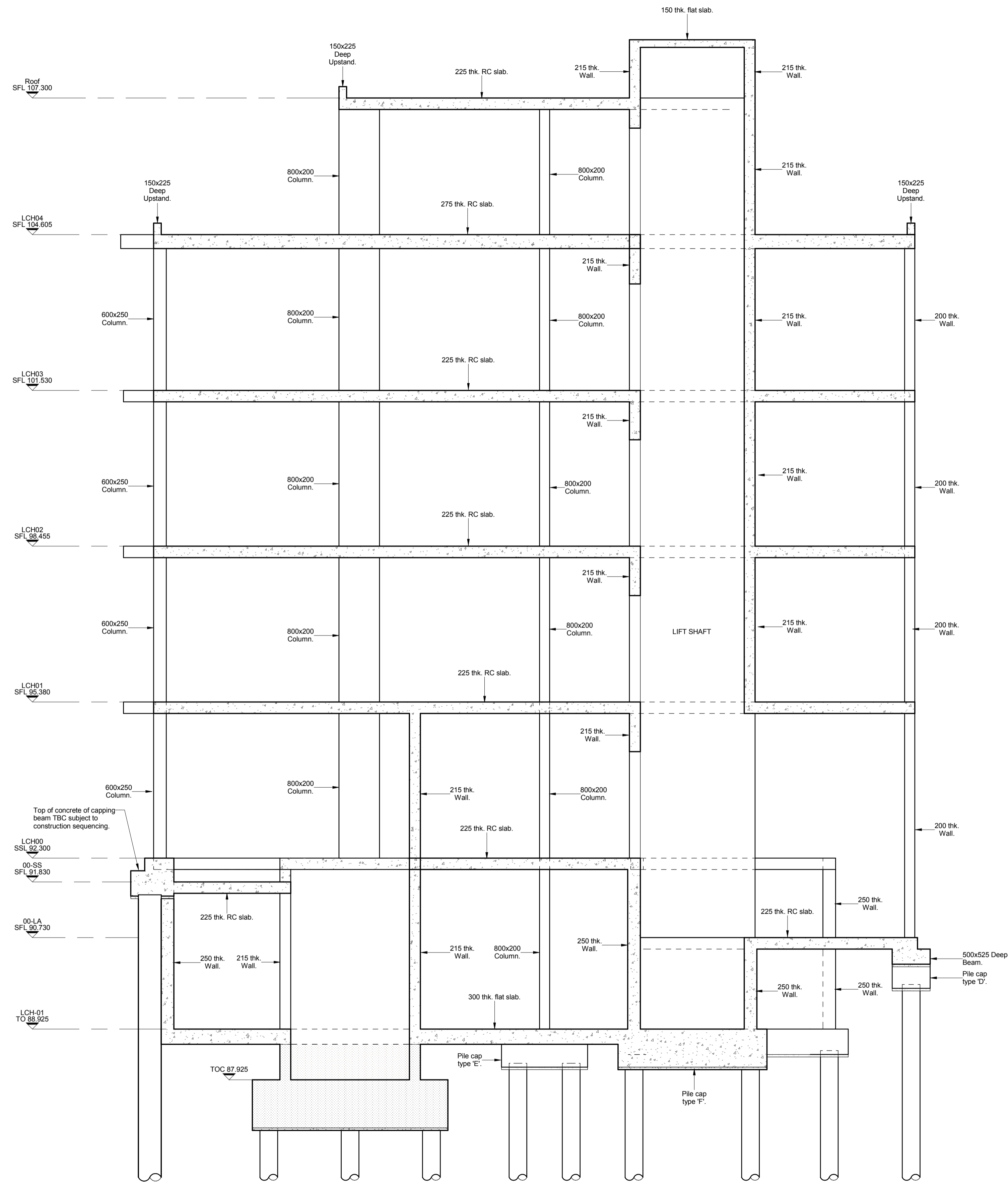
Section A-A scale 1 : 50
