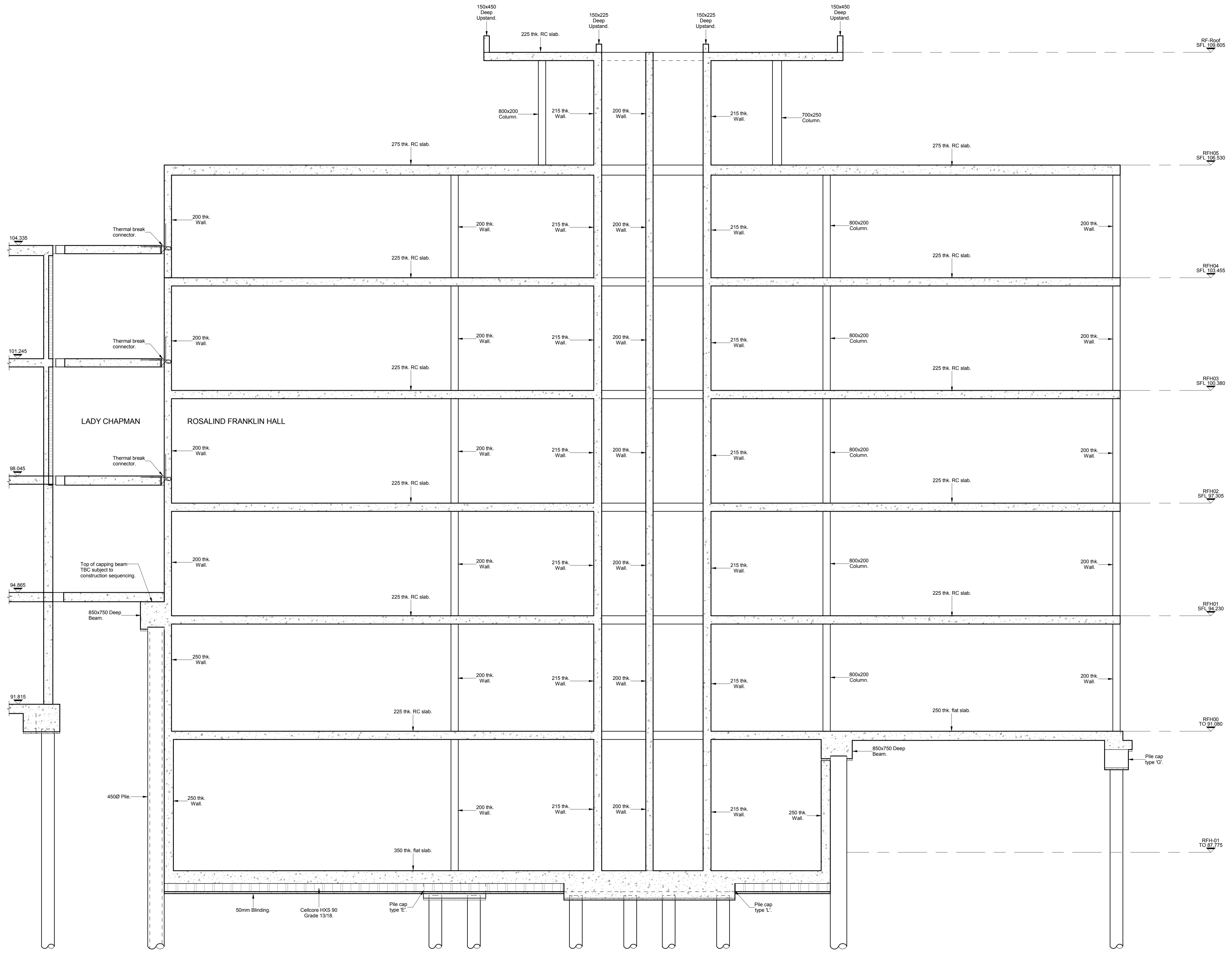
A | Section A-A scale 1 : 50
