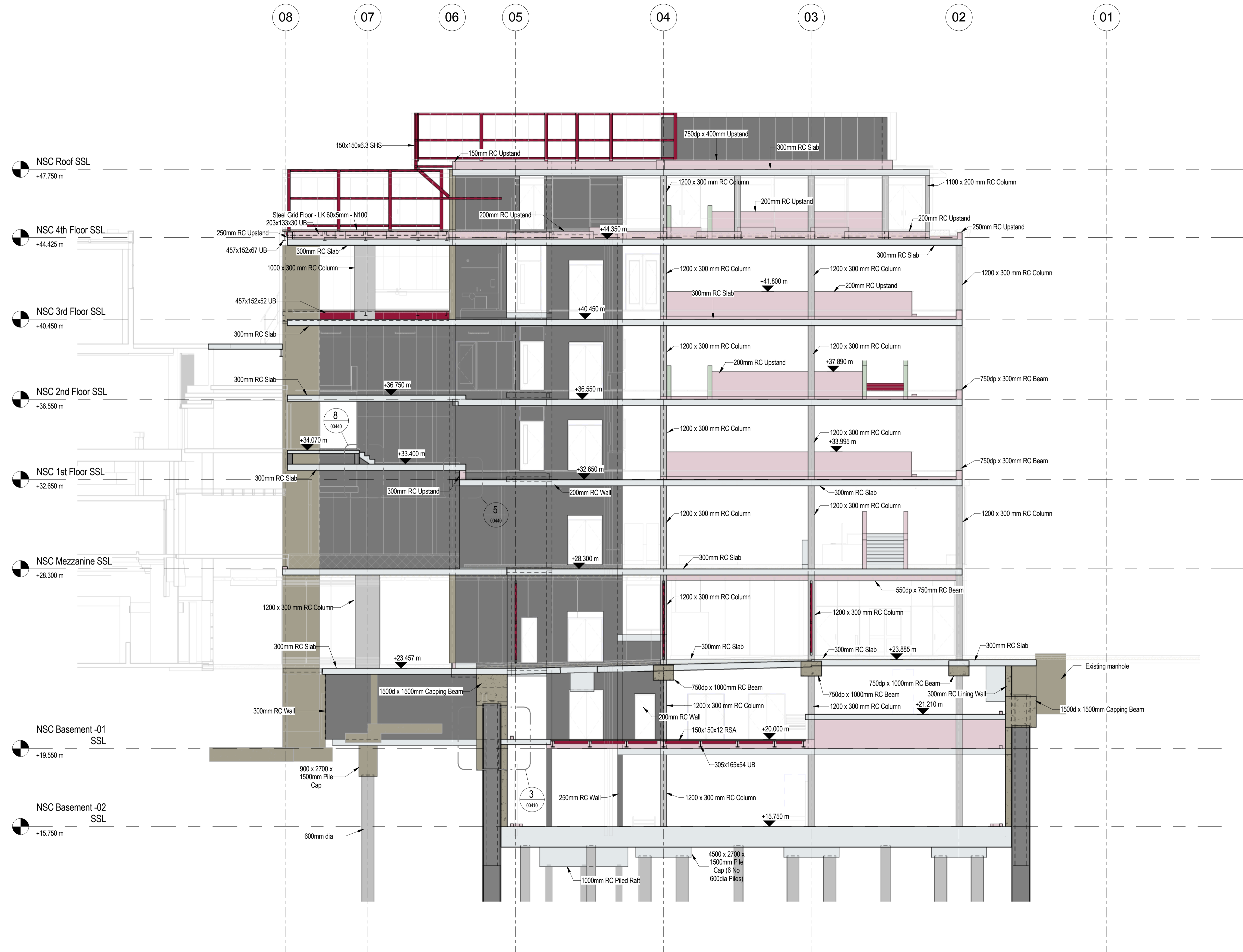
SECTION JJ 1 : 100
