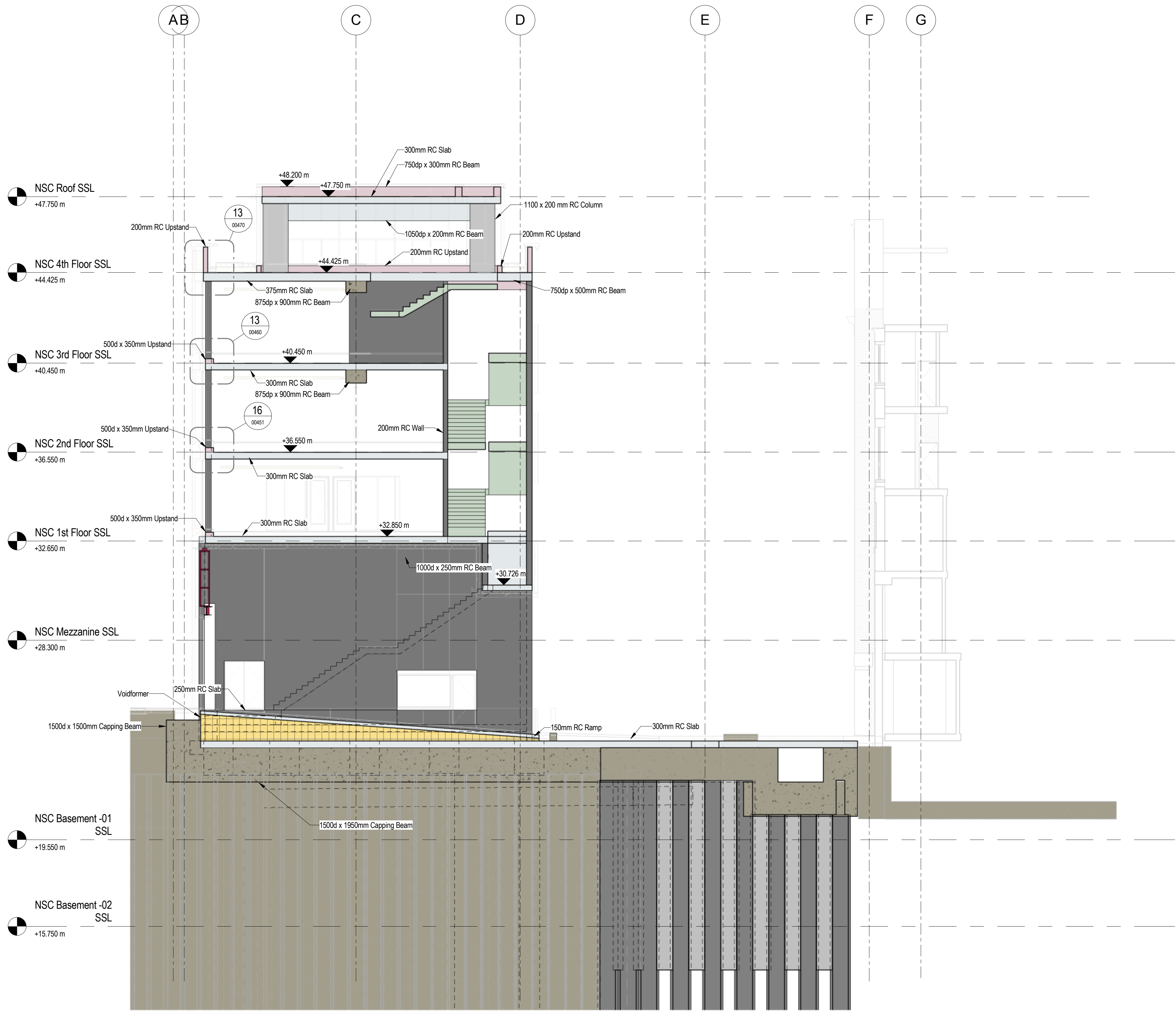
SECTION GG 1 : 100
