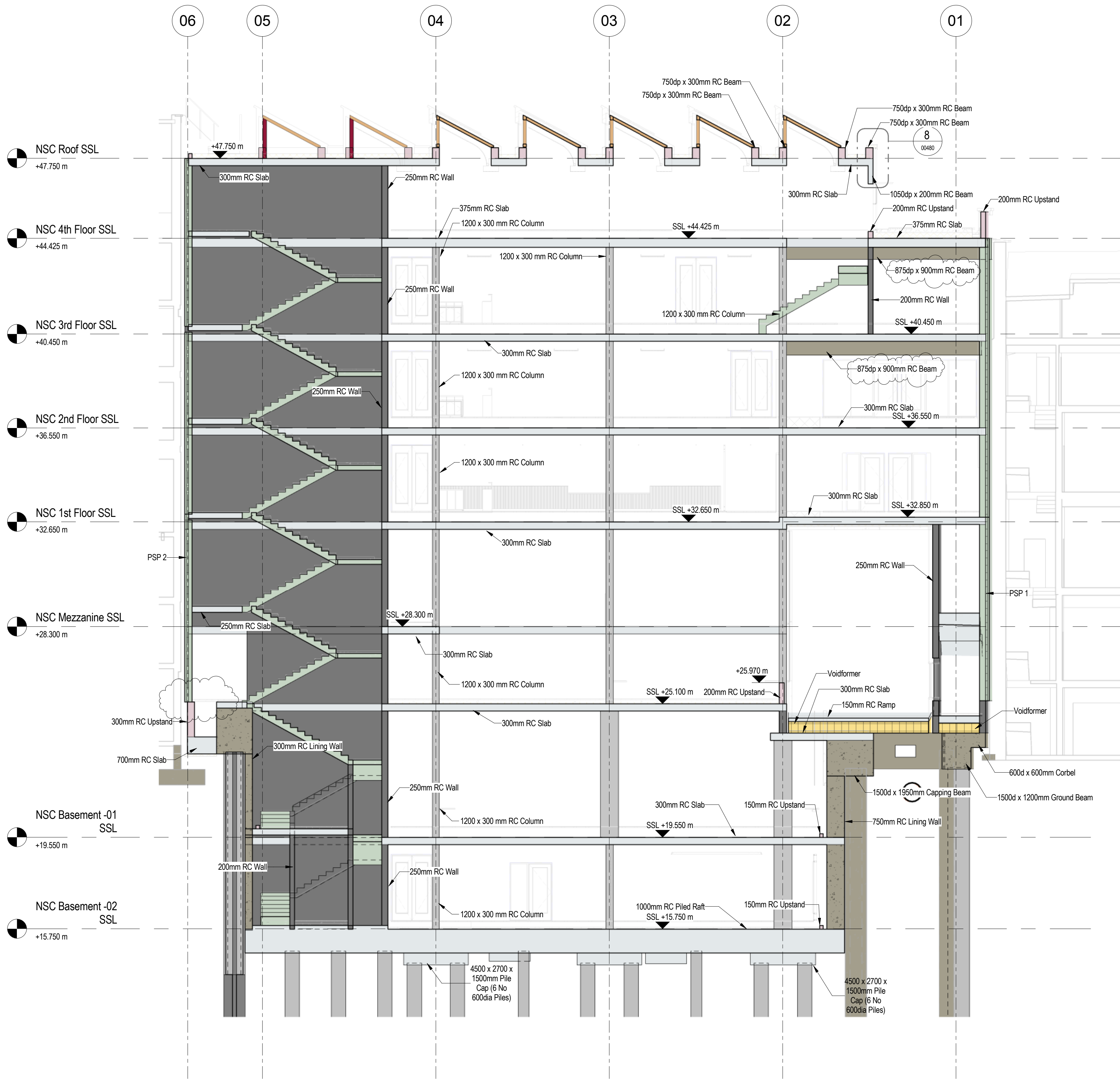
DD SECTION DD 1 : 100
