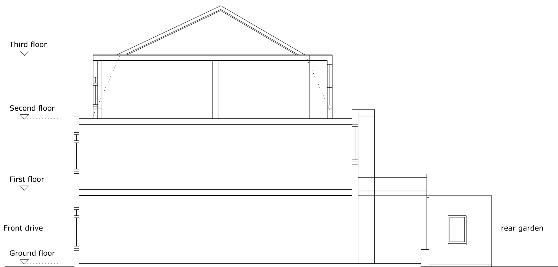
Section A-A
