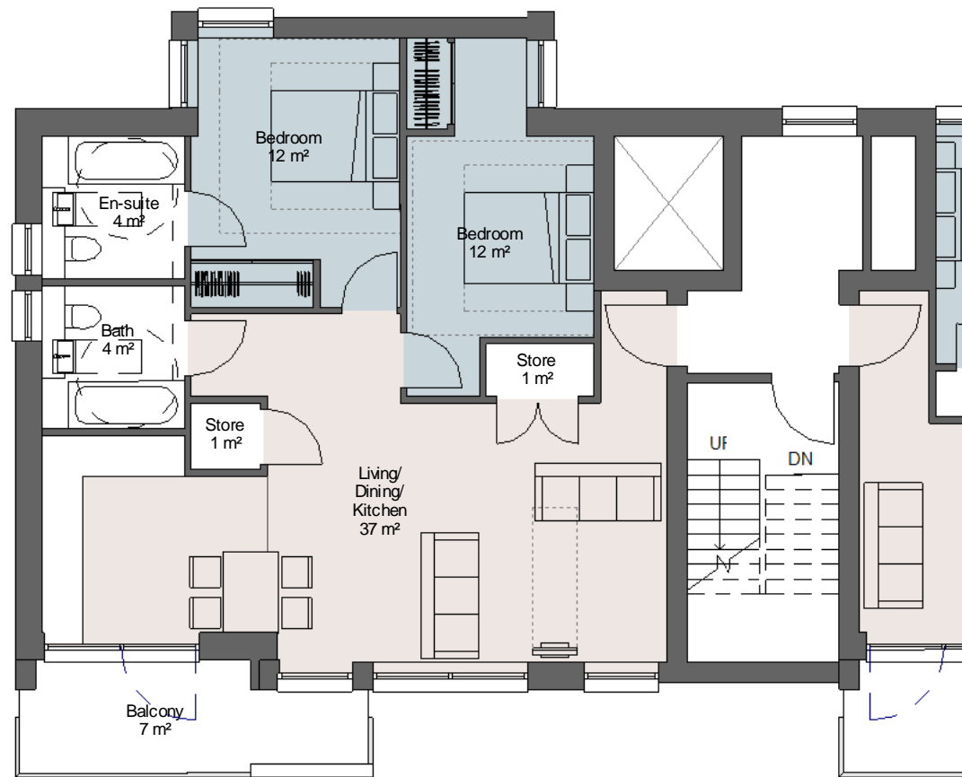
1 Private - Type PN - 2B4P 1 : 100 GIA - 75m²
