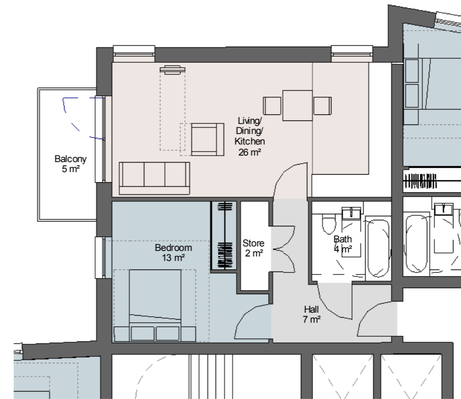
2 Private - Type PU - 1B2P 1 : 100 GIA - 56m²
