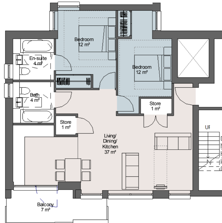
1 Private - Type PN - 2B4P 1 : 100 GIA - 75m²
