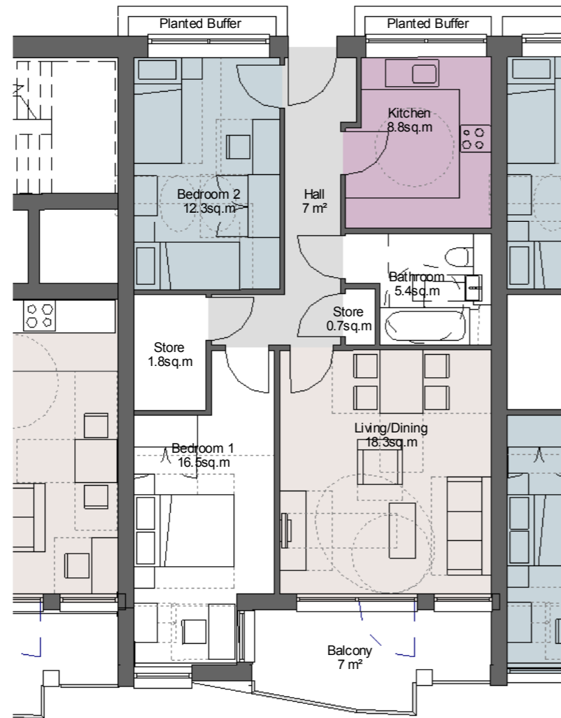
1 Affordable - Type AI - 2B4P 1 : 100 GIA - 73m²
