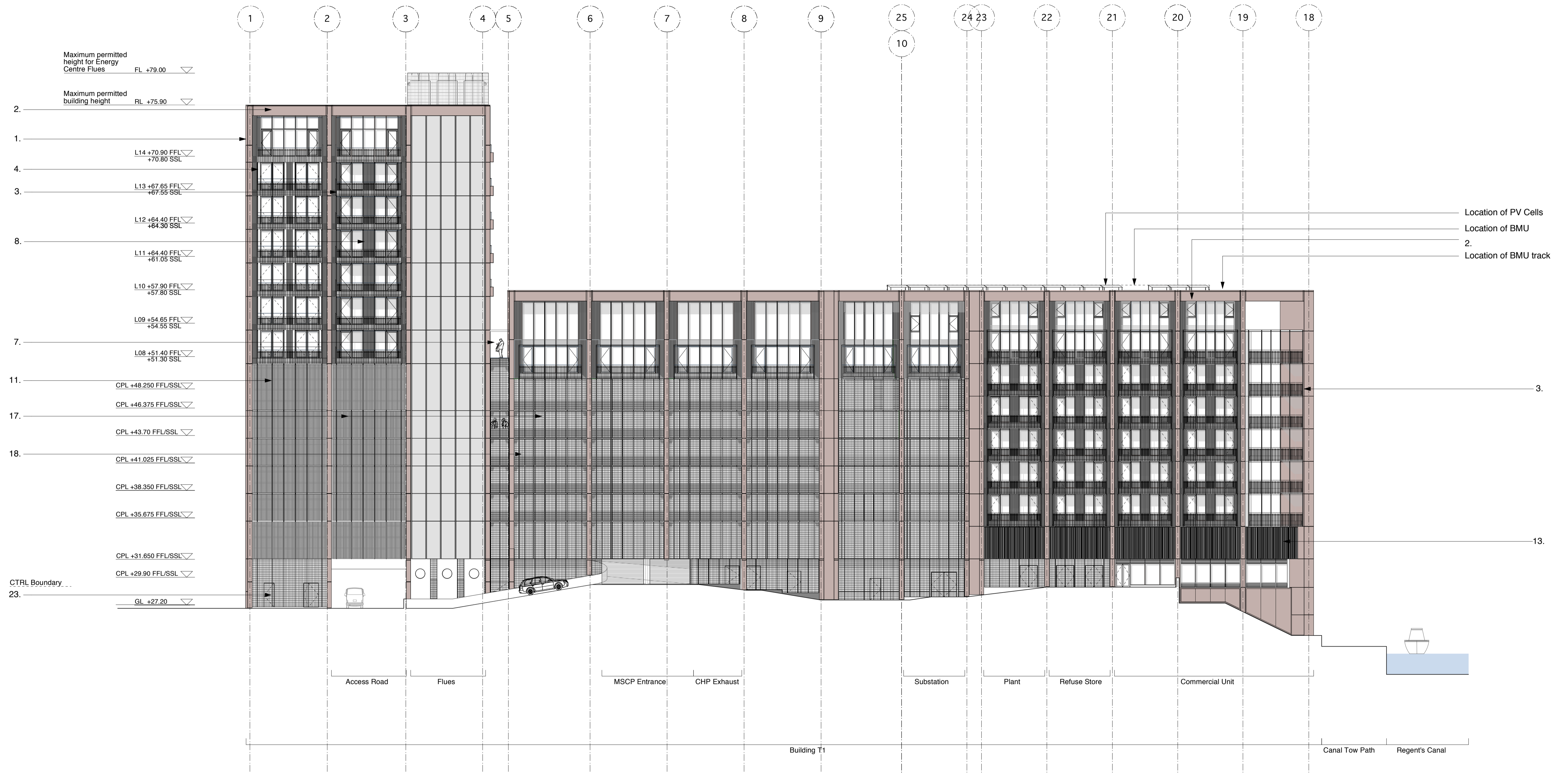
1 West Elevation Scale: 1:200
