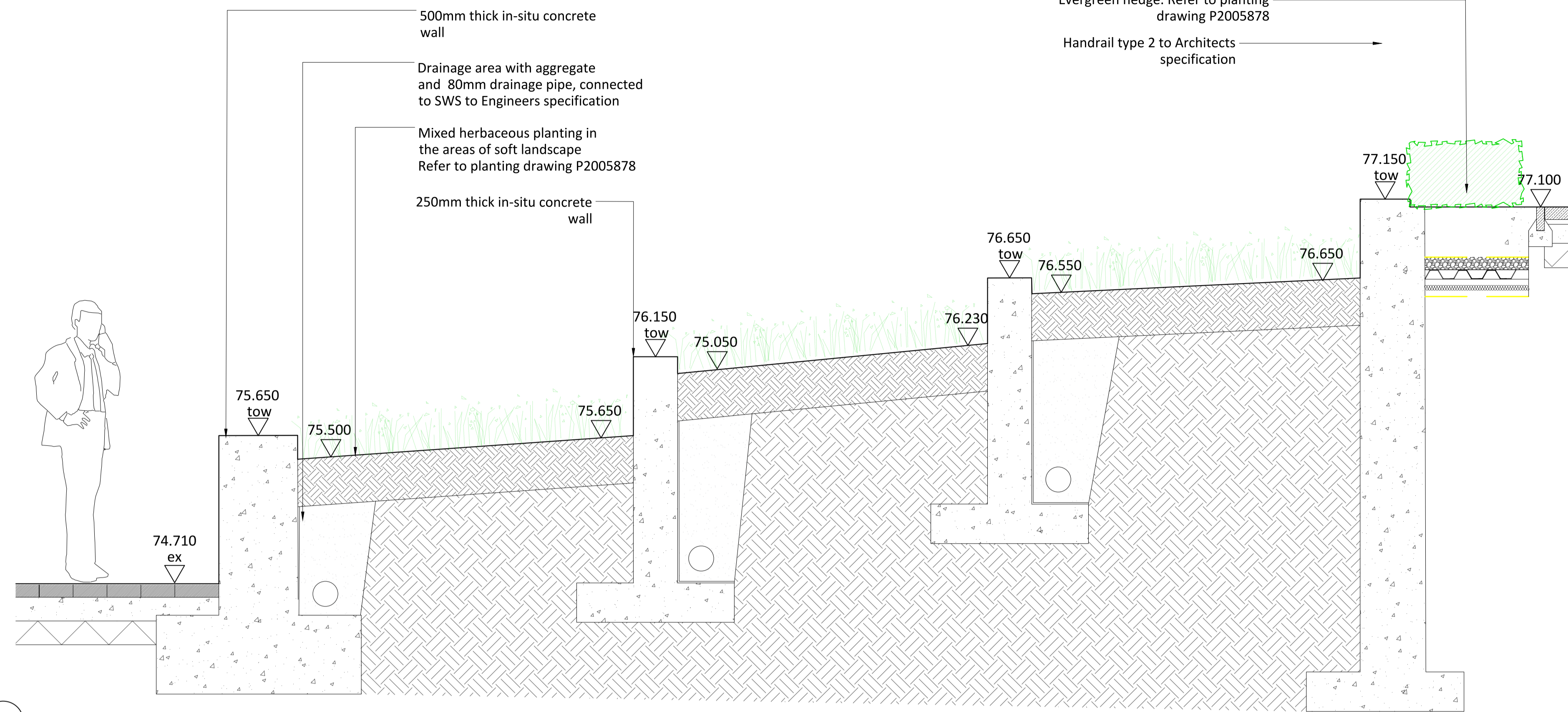
E Scale 1:20
